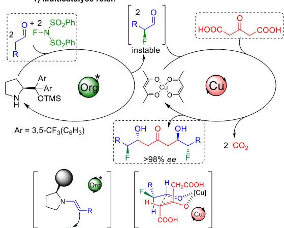
Figure 2 – Exemple de multicatylse relais
