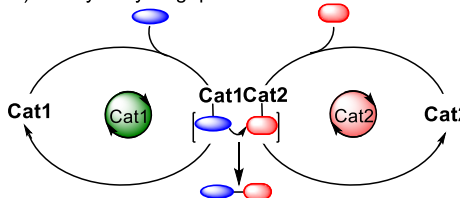
Figure 1 –Principes des réactions multicatalysées
