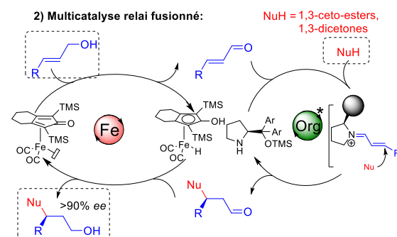
Figure 3 – Cycles catalytiques relais fusionnés
