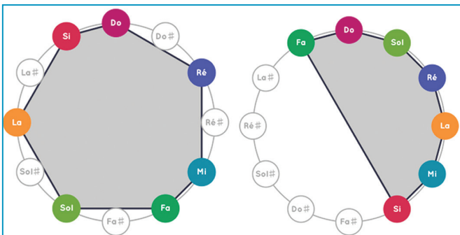
Fig. 4 : La gamme diatonique dans le cercle chromatique (à gauche) et dans la représentation circulaire associée au cycle des quintes (à droite).
