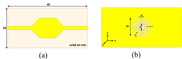
Fig. 2. Topologie de la structure du capteur microondes (a) Ligne d'alimentation élargie (b) Plan de masse gravé avec le CSRR
