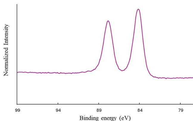
Fig. 5. : XPS Au 4 f peaks for Au/ZrO 2 catalyst.
