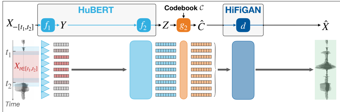
(d) HuBERT-based inpainting pipeline – blind case (inference)
