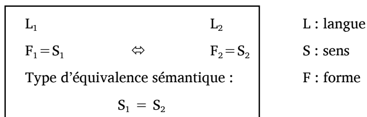
Schéma 1. Équivalence sémantique S_1 = S_2
