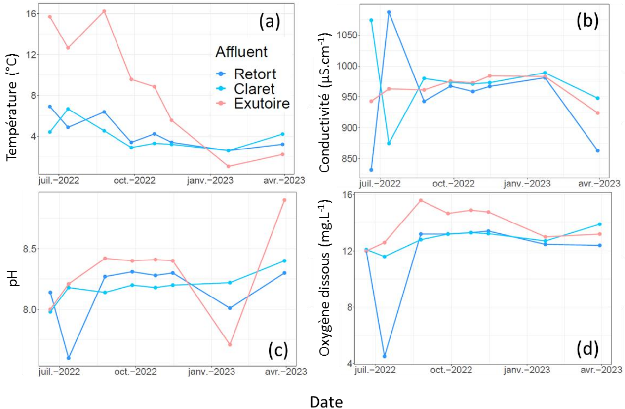
Figure 22. Evolution de la température (°C) (a), de la conductivité ( \mu\text{S}\cdot\text{cm}^{-1} ) (b), du pH (c) et de la concentration en oxygène dissous ( \text{mg}\cdot\text{L}^{-1} ) (d) des deux principaux tributaires et de l'exutoire, mesurés au niveau des stations 3,4 & 5 de juin 2022 à Mars 2023 (une mesure par mois).
