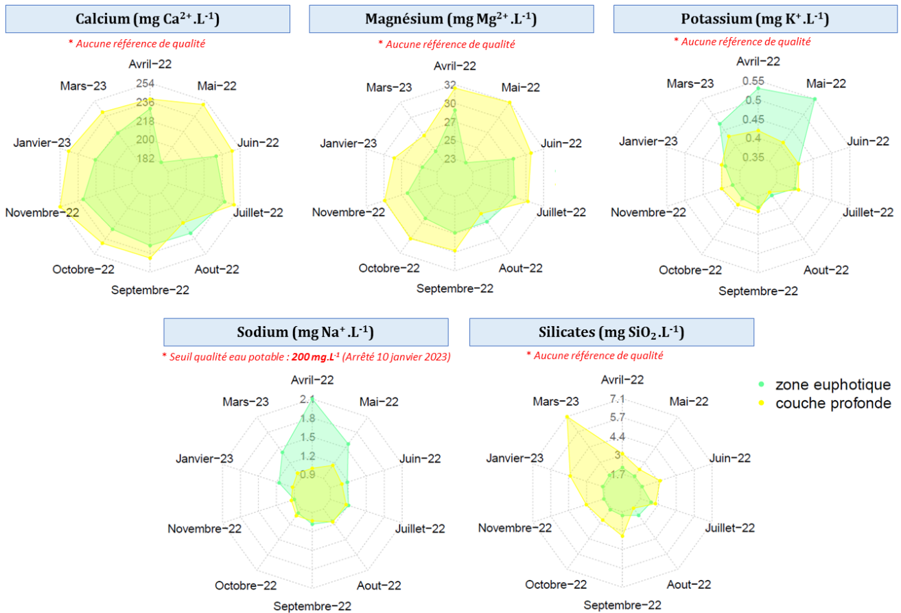
Figure 16. Mesures des concentrations en calcium (mg Ca 2+ .L-1), magnésium (mg Mg 2+ .L-1), potassium (mg K + .L-1), sodium (mg Na + .L-1) et silicates (mgSiO 2 .L-1) au niveau de la Station 2 (côté exutoire), dans le Lac de Tignes, d'Avril 2022 à Mars 2023.
