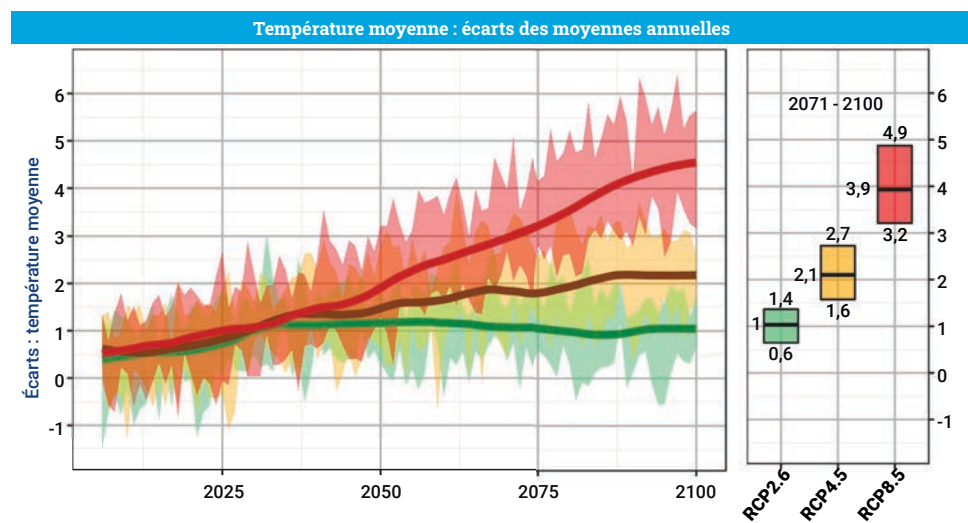
Figure 12 : Évolution de l'écart de température moyenne annuelle au cours du XXI e siècle (par rapport à la référence 1976-2005) pour les trois scénarios RCP2.6 en vert, RCP4.5 en orange et RCP8.5 en rouge. Le trait continu correspond à la médiane lissée (moyenne glissante sur 20 ans). L'enveloppe de couleur illustre l'intervalle entre les centiles 5 et 95 de la distribution de l'ensemble des simulations. La boxplot de droite représente les écarts de température sur le dernier horizon temporel (2071-2100).
