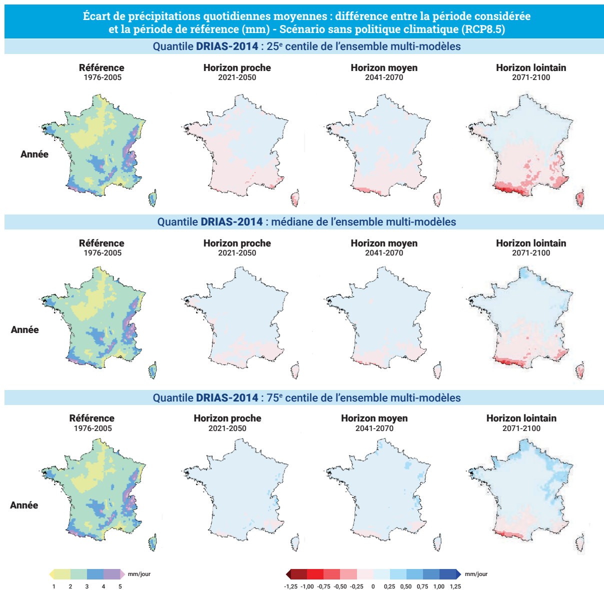
Figure F6.6 : La colonne de gauche représente la climatologie de référence (1976-2005) pour des précipitations annuelles. Le reste du panel de cartes correspond aux écarts des précipitations annuelles par rapport à la référence pour le scénario RCP8.5, en colonne les différents horizons (H1, H2, H3) et en ligne les produits de distribution de l'ensemble DRIAS-2014 (25 e , 50 e et 75 e centiles).
