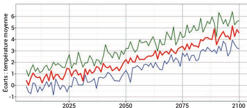
Température moyenne : écarts des moyennes annuelles du RCP8.5
