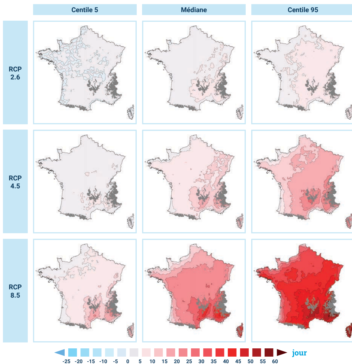
Figure 21 : Cartes des écarts de nombre de jours de vagues de chaleur à l'horizon fin de siècle pour les trois RCP et selon les paramètres de la distribution C5, C50 et C95.
