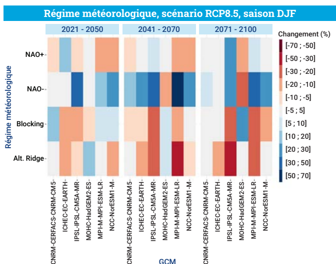
Figures F4.1 : Évolution relative de la fréquence des régimes en hiver pour les 6 GCM utilisés comme GCM forceur dans le jeu DRIAS-2020 selon les horizons temporels : haut RCP2.6, milieu RCP4.5, bas RCP8.5.
