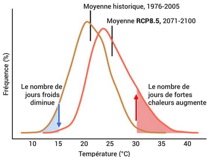
Figure F5.1 : Distributions statistiques des températures quotidiennes en conditions climatiques actuelles (marron) et futures (rouge). Les extrêmes sont définis aux extrémités de la distribution comme des événements dépassant un certain seuil (zones colorées). Un déplacement ou un changement de la distribution dans le temps, entraîne des changements dans l'occurrence des extrêmes. Les surfaces sous les courbes sont proportionnelles à la probabilité d'occurrence.
