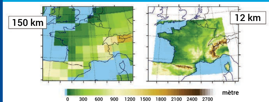
Figure B1 : Illustration de la différence de résolution entre la modélisation climatique globale (150 km de résolution) et la modélisation climatique régionale (12 km) sur le relief et le trait de côte de la France (C. Cassou, Cerfacs). L'échelle de couleur représente l'altitude des mailles des modèles (en mètres).
