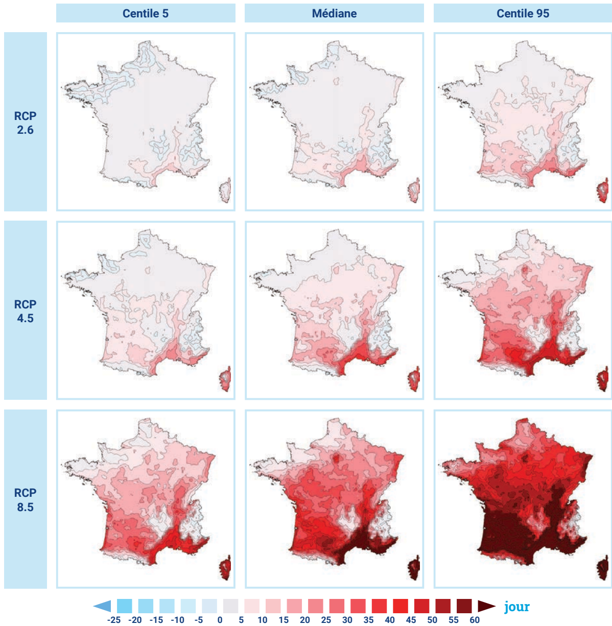
Figure 23 : Cartes des écarts de nombre de nuits tropicales à l'horizon fin de siècle pour les trois RCP et selon les paramètres de la distribution C5, C50 et C95.
