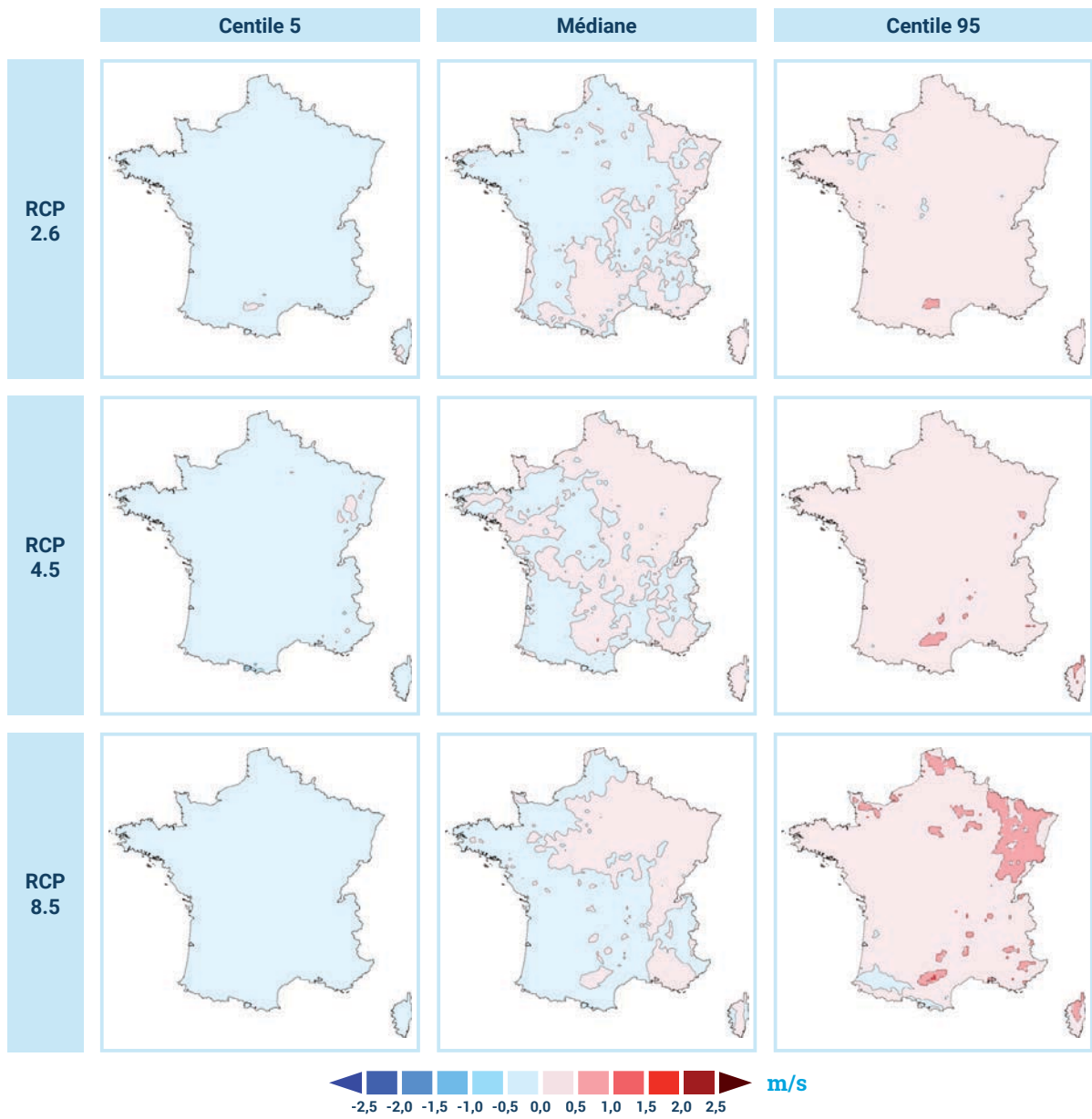
Figure 33 : Cartes des écarts de l'intensité des vents forts pour les trois RCP et l'horizon fin de siècle, selon les paramètres de la distribution C5, C50 et C95.
