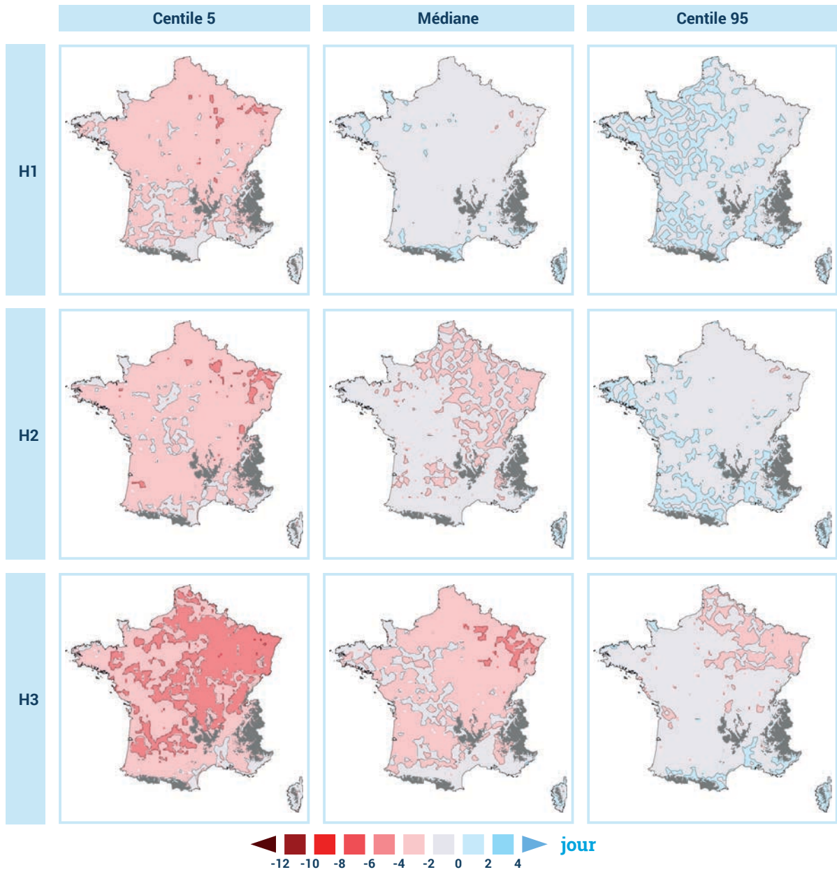
Figure 24 : Cartes des écarts de nombre de jours de vagues de froid pour le RCP8.5 et les trois horizons et selon les paramètres de la distribution C5, C50 et C95.
