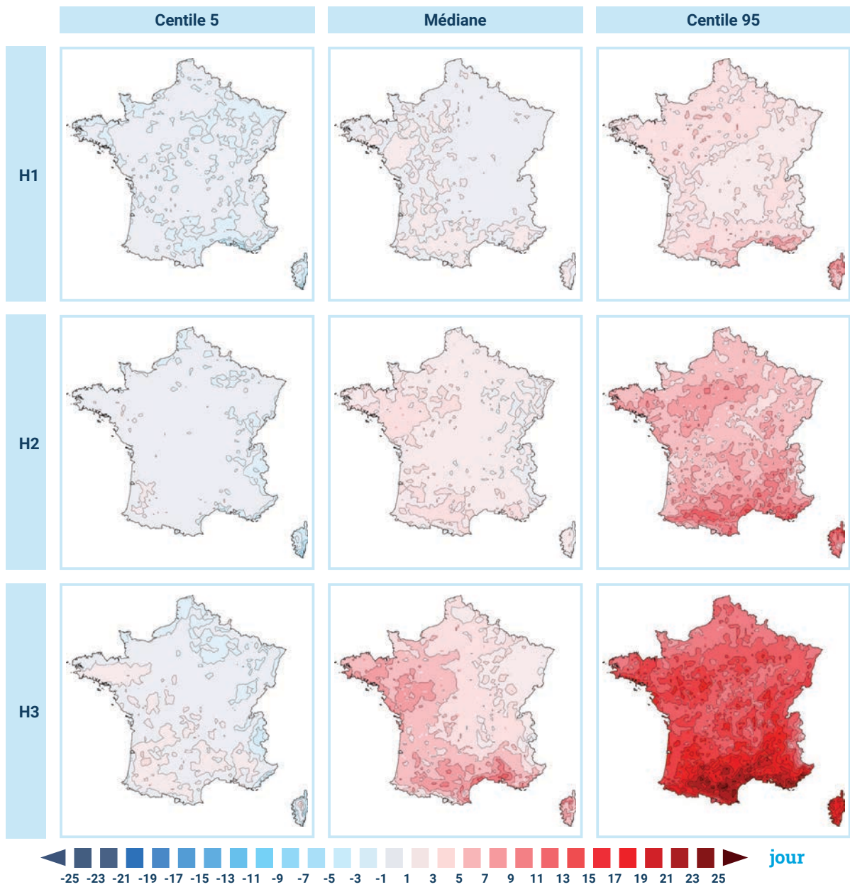
Figure 30 : Cartes des écarts du nombre maximum de jours secs consécutifs en été pour le RCP8.5 et les trois horizons et les trois horizons selon les paramètres de la distribution C5, C50 et C95.
