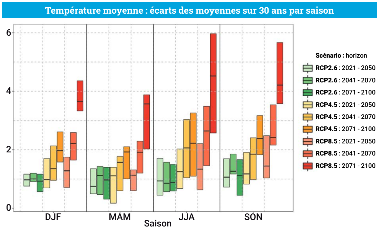
Figure 15 : Graphique de l'évolution saisonnière des écarts de températures par RCP et horizon temporel.
