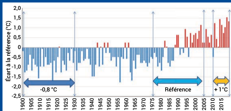
Figure C1 : Evolution de l'anomalie de température moyenne annuelle en France de 1900 à 2019 par rapport à la période de référence 1976-2005. La décennie actuelle (2011-2019) est plus chaude (+1°C) que la période de référence 1976-2005, elle-même déjà réchauffée (+0,8°C) par rapport au début du XX e siècle (période 1901-1930).
