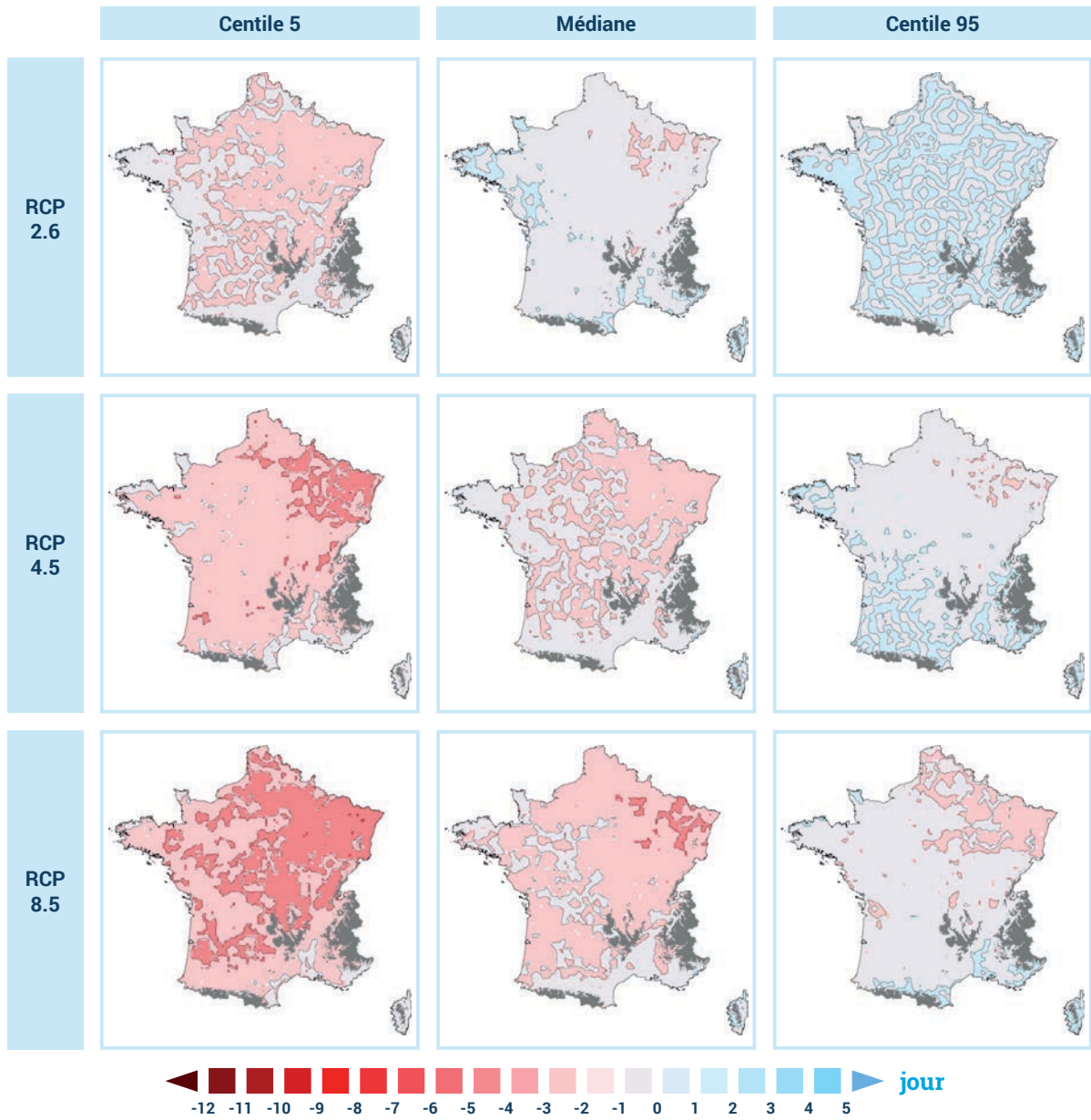
Figure 25 : Cartes des écarts de nombre de jours de vagues de froid à l'horizon fin de siècle pour les trois RCP et selon les paramètres de la distribution C5, C50 et C95.
