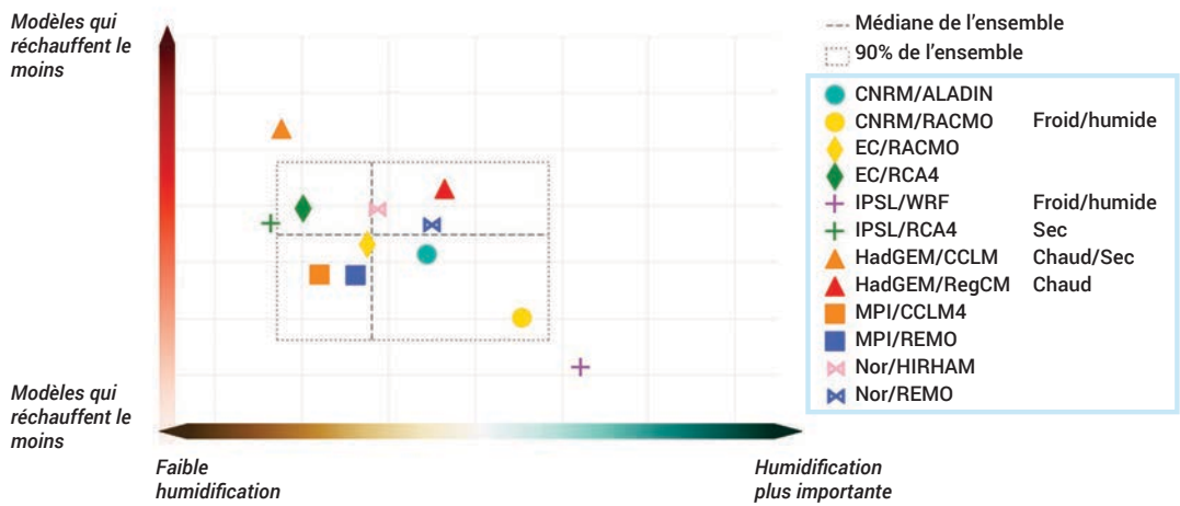
Figure 7 : Dispersion des simulations individuelles de l'ensemble DRIAS-2020 selon les évolutions prévues de précipitation (abscisses) et température (ordonnées) pour un scénario RCP8.5 à l'horizon fin de siècle et deux saisons : hiver en haut, été en bas.
