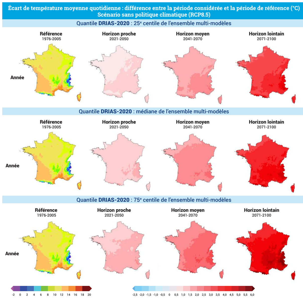
Figure F6.2 : La colonne de gauche représente la climatologie de référence (1976-2005) pour les températures annuelles. Le reste du panel de cartes correspond aux écarts de températures annuelles par rapport à la référence pour le scénario RCP8.5, en colonne les différents horizons (H1, H2, H3) et en ligne les produits de distribution de l'ensemble DRIAS-2020 (25 e , 50 e et 75 e centiles).
