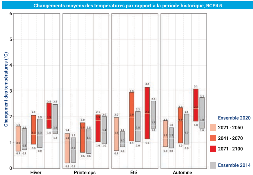
Figures F6.4 : Représentation sous forme de boxplot des écarts des températures saisonnières des jeux DRIAS-2014 et DRIAS-2020 par rapport à la référence (1976-2005). Les boîtes représentent les 5 e et 95 e centiles et la barre blanche la médiane (en haut pour le scénario d'émission RCP8.5 et en bas pour le RCP4.5).
