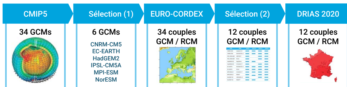
Figure 6 : Synthèse de l'ensemble des étapes de la sélection des simulations pour le jeu DRIAS-2020. Les 12 couples GCM/RCM sélectionnées à partir de l'ensemble Euro-Cordex ont été corrigées par la méthode statistique ADAMONT
