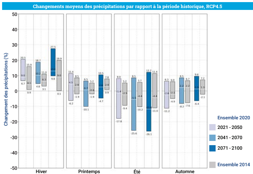
Figure F6.7 : Représentation sous forme de boxplot des écarts de précipitations saisonnières des jeux DRIAS 2014 et DRIAS 2020 par rapport à la référence (1976-2005). Les boîtes représentent les 5 e -95 e centiles et la barre blanche la médiane (en haut pour le scénario d'émission RCP8.5 et en bas pour le RCP4.5).
