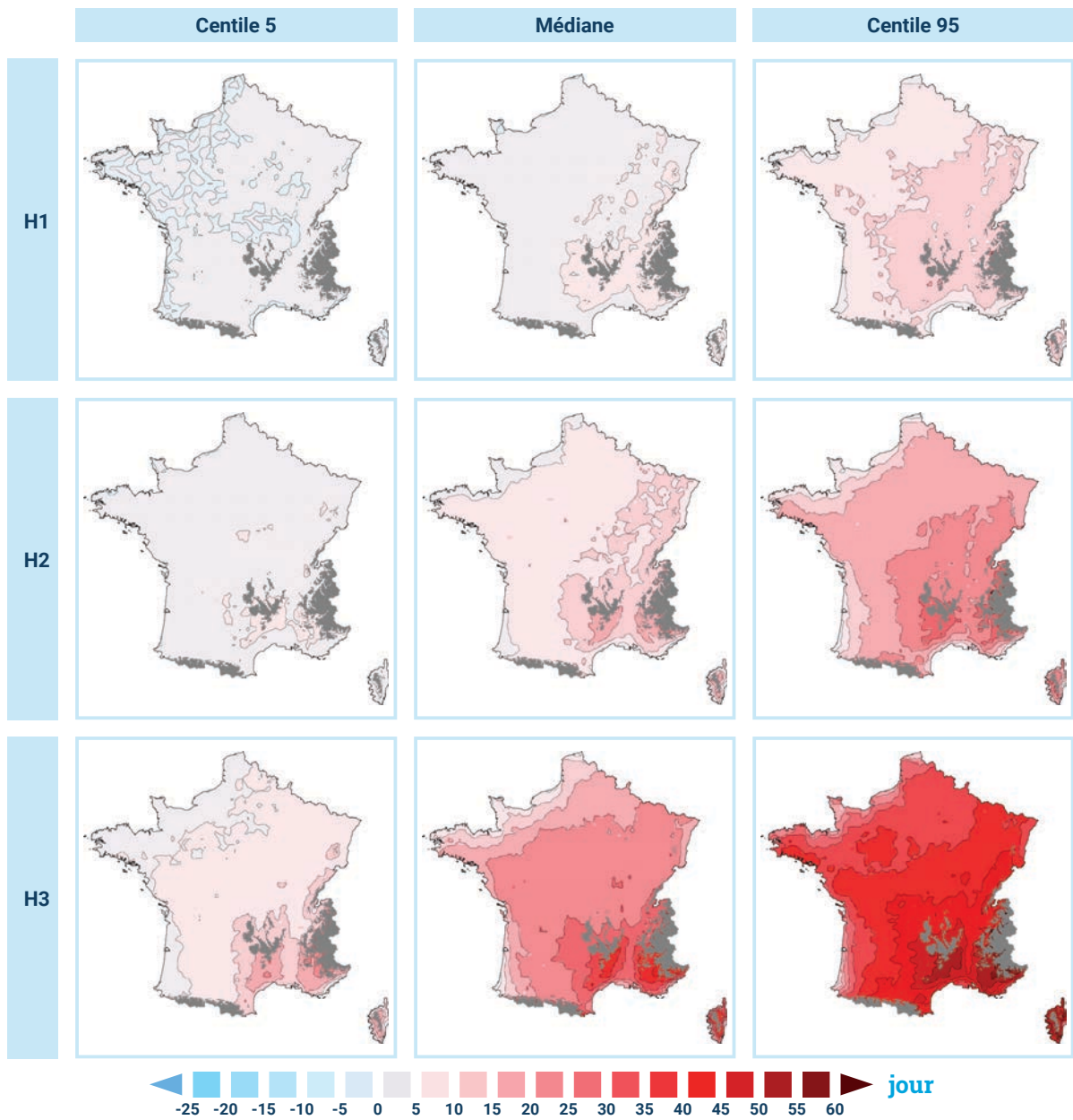
Figure 20 : Cartes des écarts de nombre de jours de vagues de chaleur pour le scénario RCP8.5 par horizon temporel et selon les paramètres de la distribution C5, C50 et C95.
