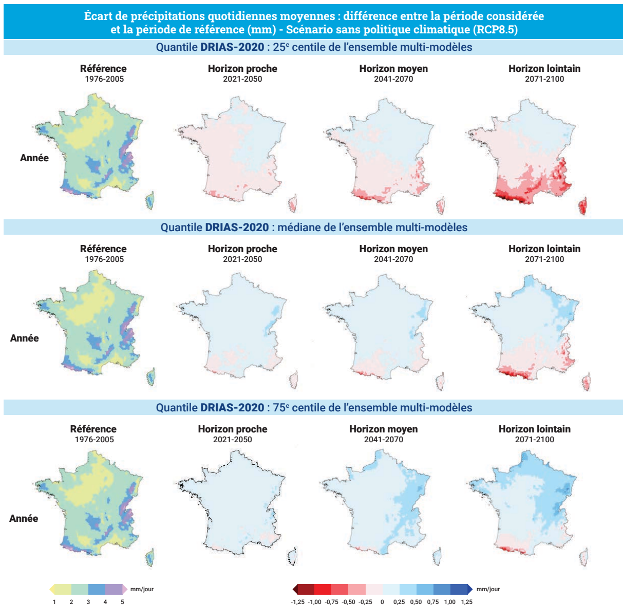
Figure F6.5 : La colonne de gauche représente la climatologie de référence (1976-2005) pour des précipitations annuelles. Le reste du panel de cartes correspond aux écarts des précipitations annuelles par rapport à la référence pour le scénario RCP8.5, en colonne les différents horizons (H1, H2, H3) et en ligne les produits de distribution de l'ensemble DRIAS-2020 (25 e , 50 e et 75 e centiles).
