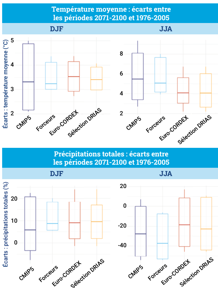
Figure 3 : Comparaison de la dispersion des simulations RCP8.5 (minimum et maximum, centiles 10, 50 et 90) issues de 4 sources de données différentes (Tous GCM de CMIP5, GCM forceurs d'Euro Cordex, ensemble Euro-Cordex, sélection DRIAS), pour 2 paramètres (température et précipitations) et 2 saisons (hiver et été).
