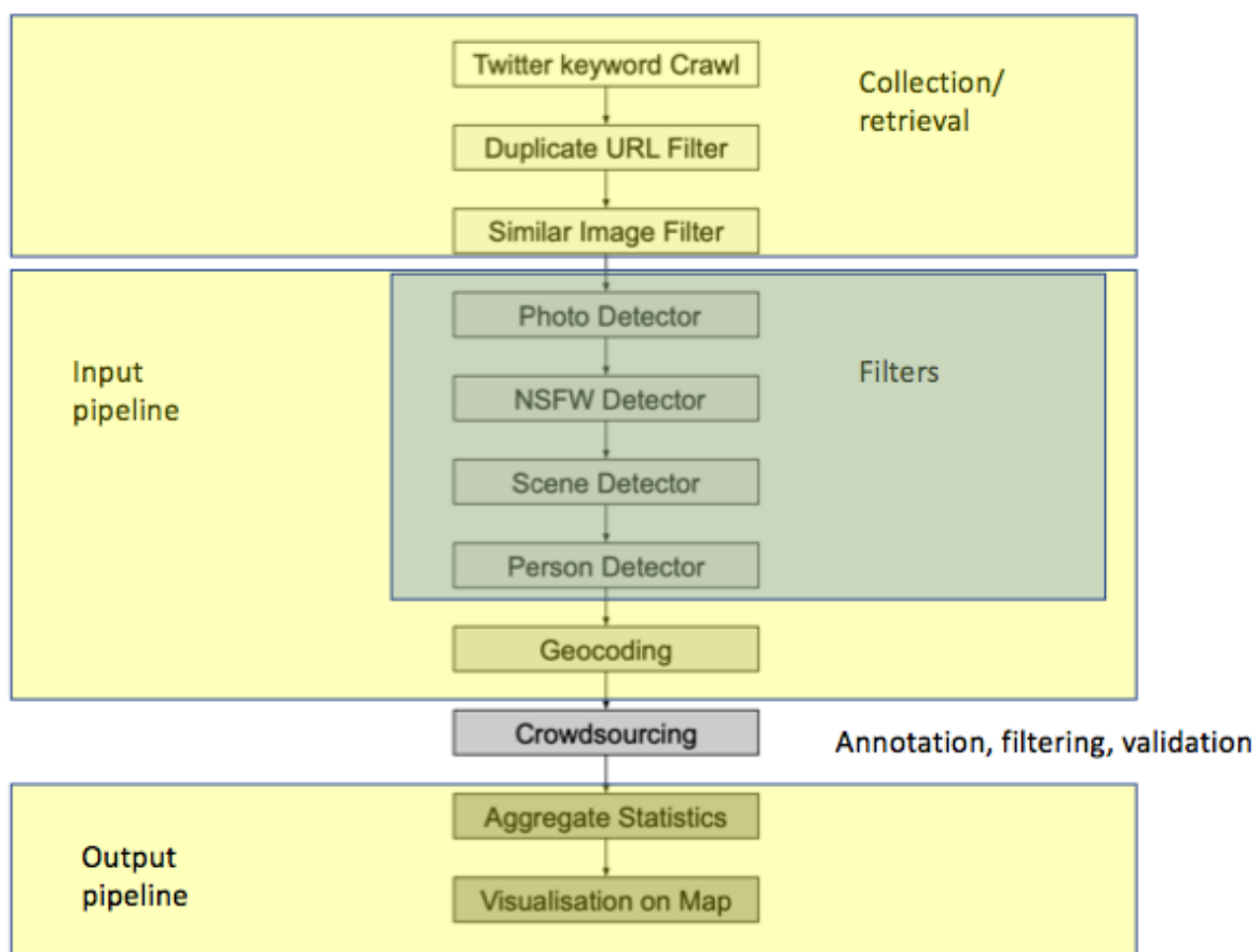
Fig. 2.5.2. VisualCit prototype pipeline
