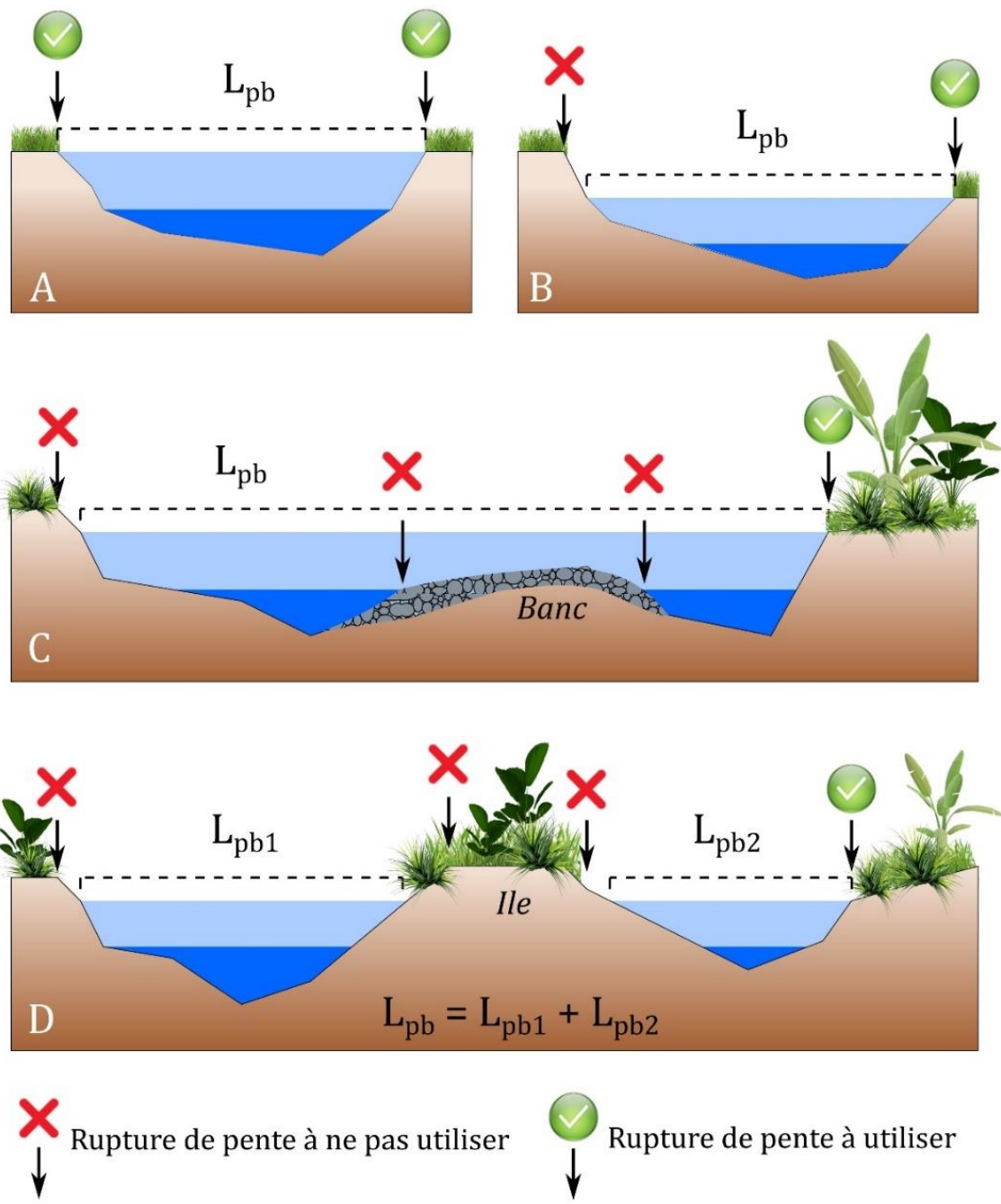
Figure 7 : Détermination de la largeur à plein bord ( L_{pb} ) (in Melun et al., 2021, d'après Baudoin et al., 2017).
