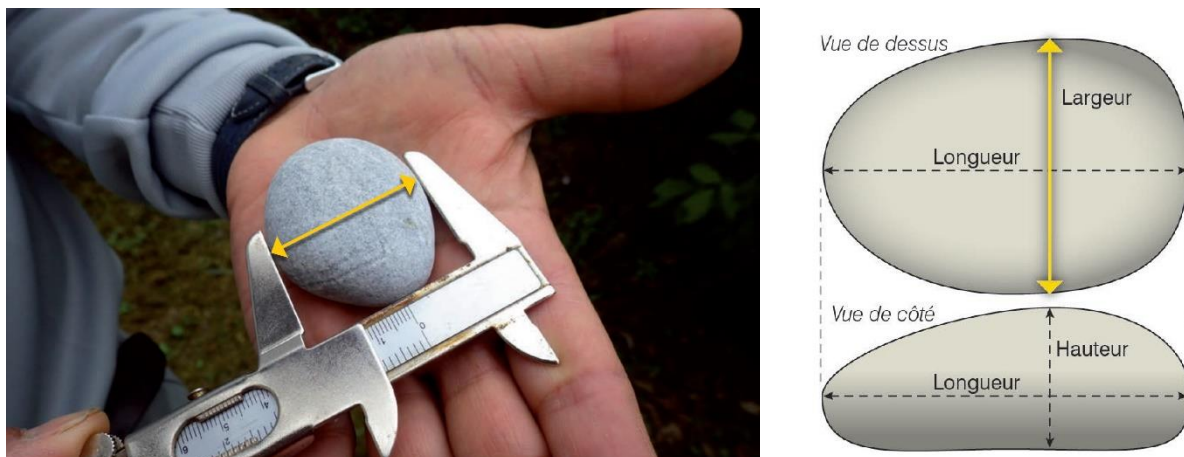
Figure 14 : Mesure de la granulométrie (in Baudoin et al., 2017).
