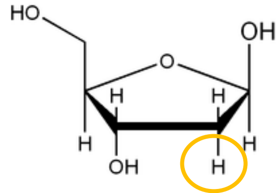
Désoxyribose = ADN
