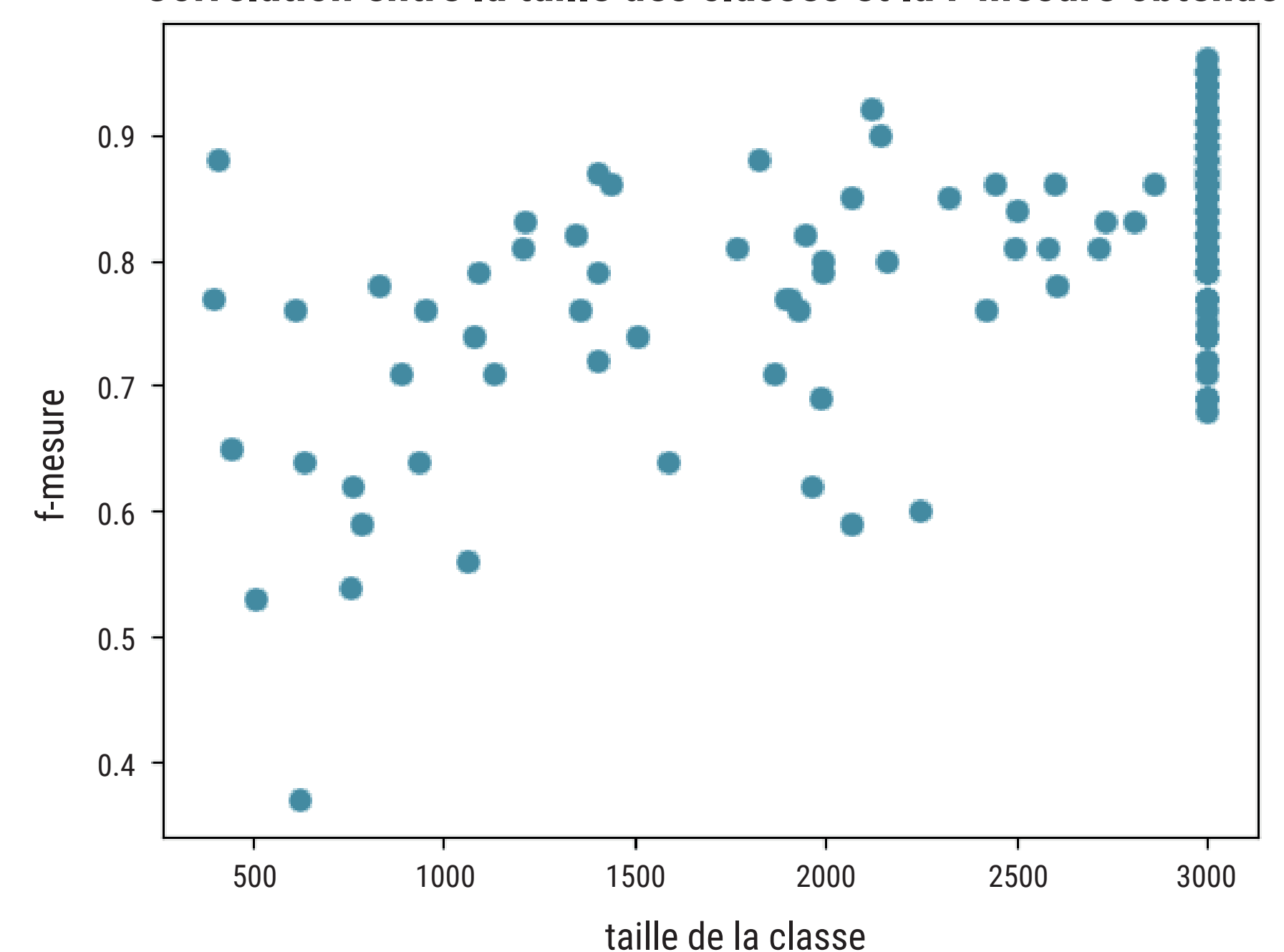
Corrélation entre la taille des classes et la f-mesure obtenue
