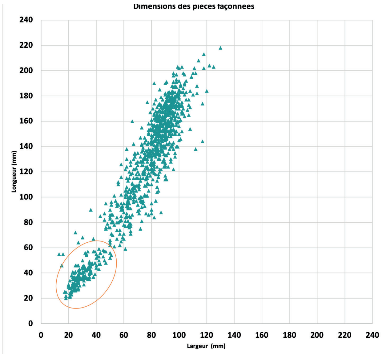
Fig. 4 – Dimensions de l'ensemble des pièces bifaciales de Garba I (n = 1002). Fig. 4 – Dimensions of the whole of the bifacial pieces (LCTs) from Garba I excavation (n=1002).
