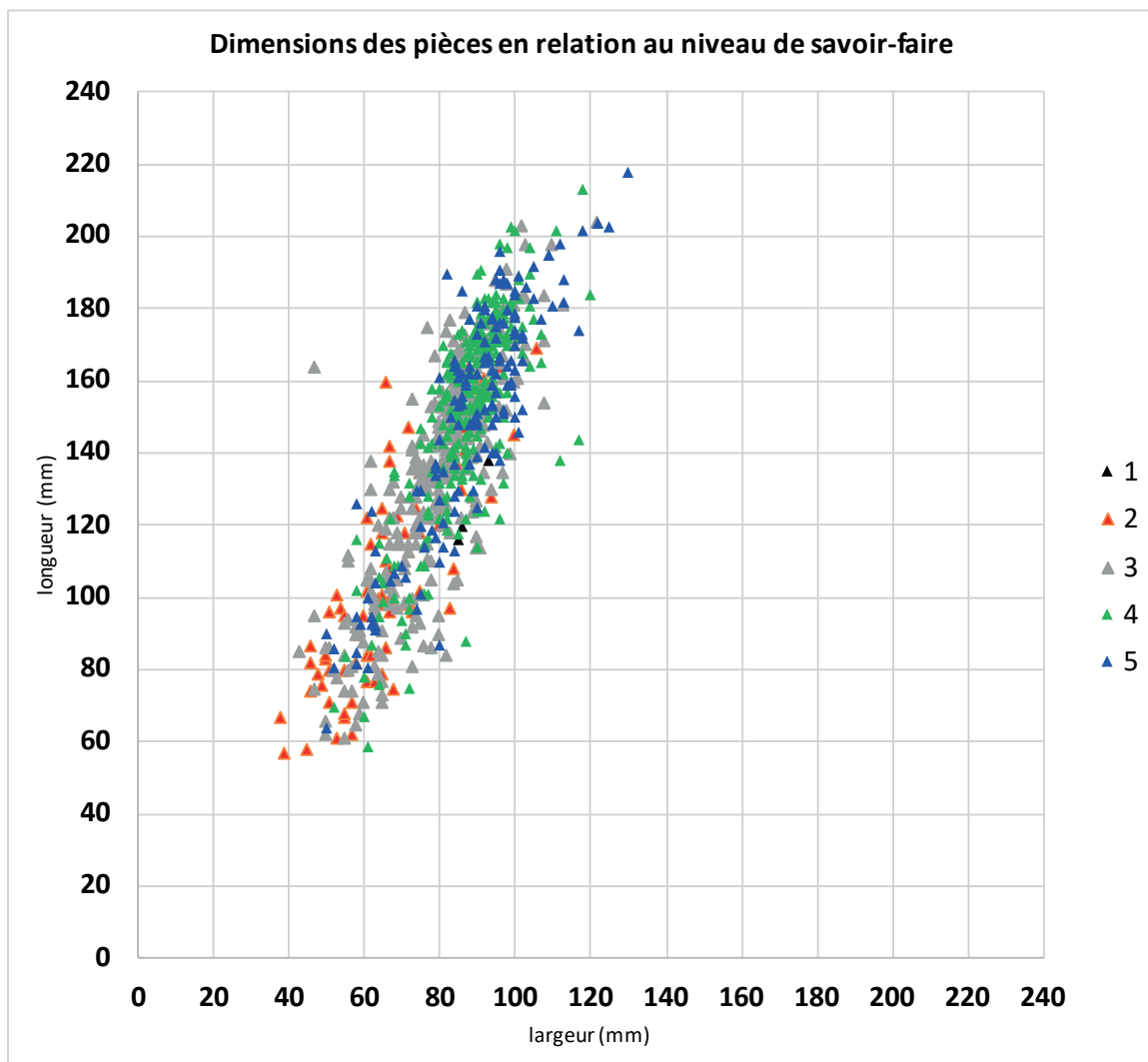
Fig. 5 – Rapport entre le niveau de savoir-faire des tailleurs et les dimensions des produits.
