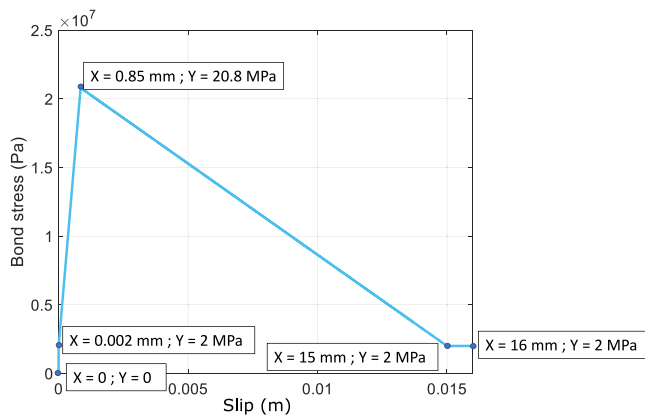
Fig. 20. Bond law.
