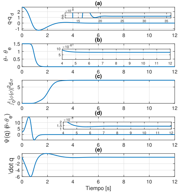
Fig. 2. Resultados de simulación del sistema de un grado de libertad con control adaptable asintótico.
