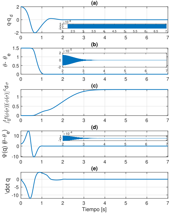
Fig. 1. Resultados de simulación del sistema de un grado de libertad con control adaptable en tiempo finito.
