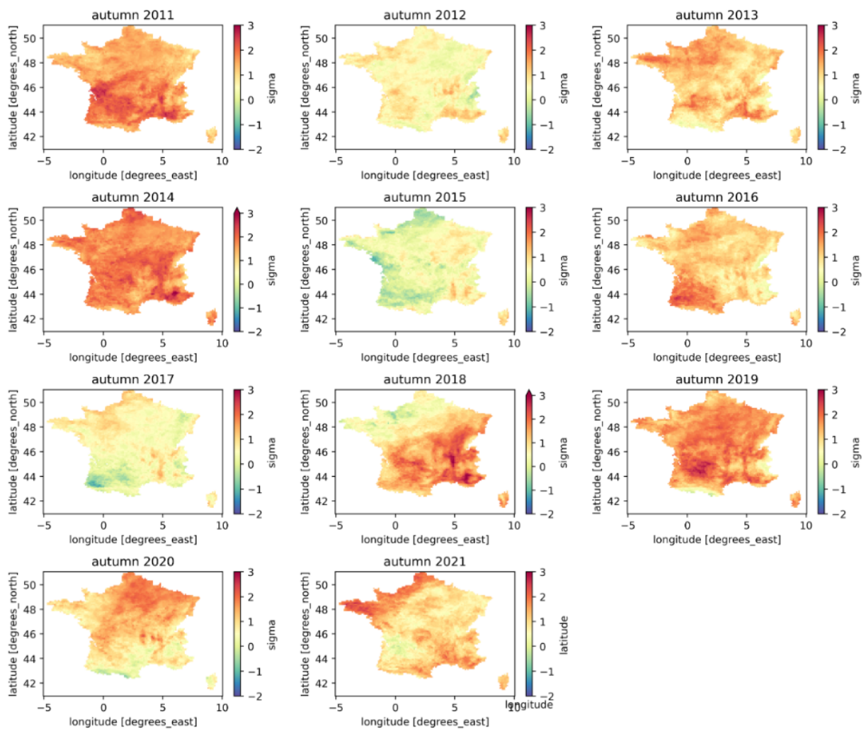
Figure A.12. Valeurs saisonnières automnales de -T10_{std} , 2011-2021.
