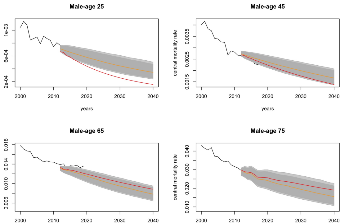
Figure 3.7. Taux de mortalité masculins projetés jusqu'en 2040, avec intervalles de confiance à 90% et 95% dans le scénario RCP2.6 (- : observé, - : prévision, - : trajectoire centrale des simulations).
