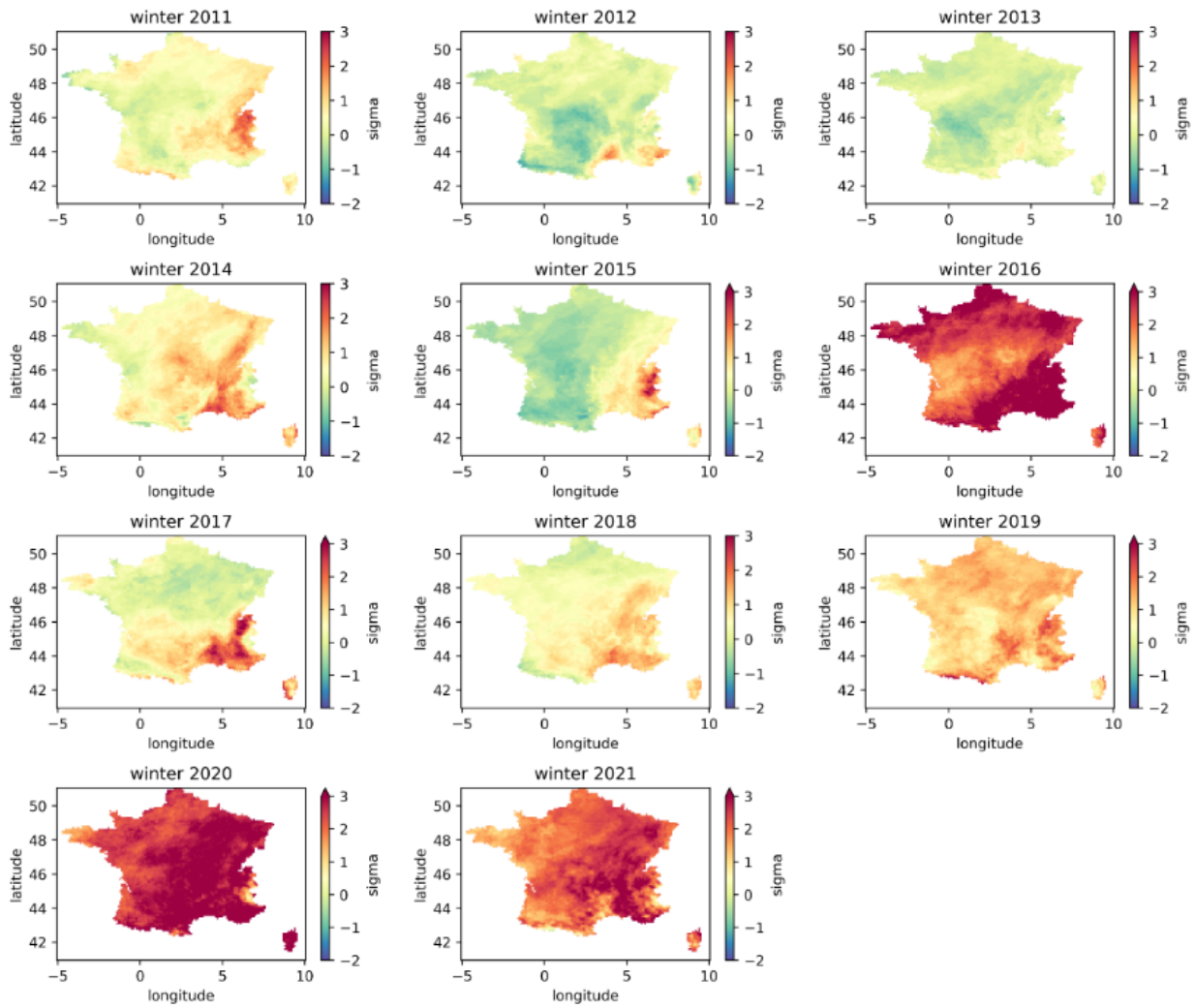
Figure A.5. Valeurs saisonnières hivernales de T90_{std} , 2011-2021.
