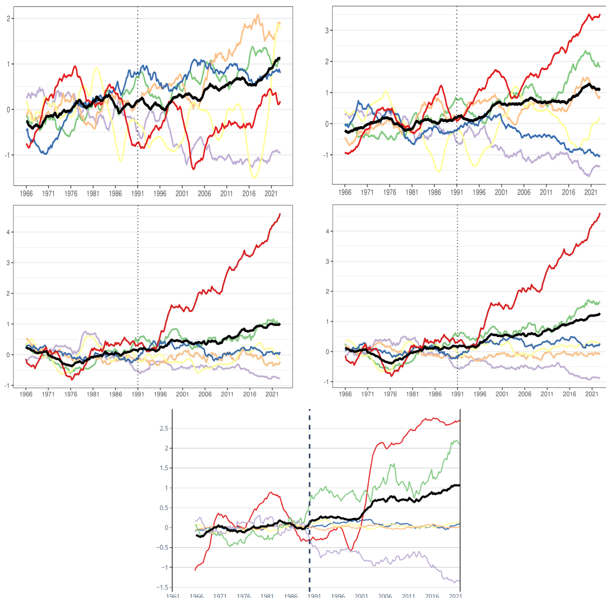
Figure 17. Moyennes mobiles saisonnières sur 5 ans des composantes d'indices actuariels climatiques (vert : T90_{std} , violet : T10_{std} , orange : P_{std} , jaune : D_{std} , bleu : W_{std} , rouge : S_{std} , noir : ACI). De haut en bas et de gauche à droite : Canada, Etats-Unis, Portugal, Espagne et France.
