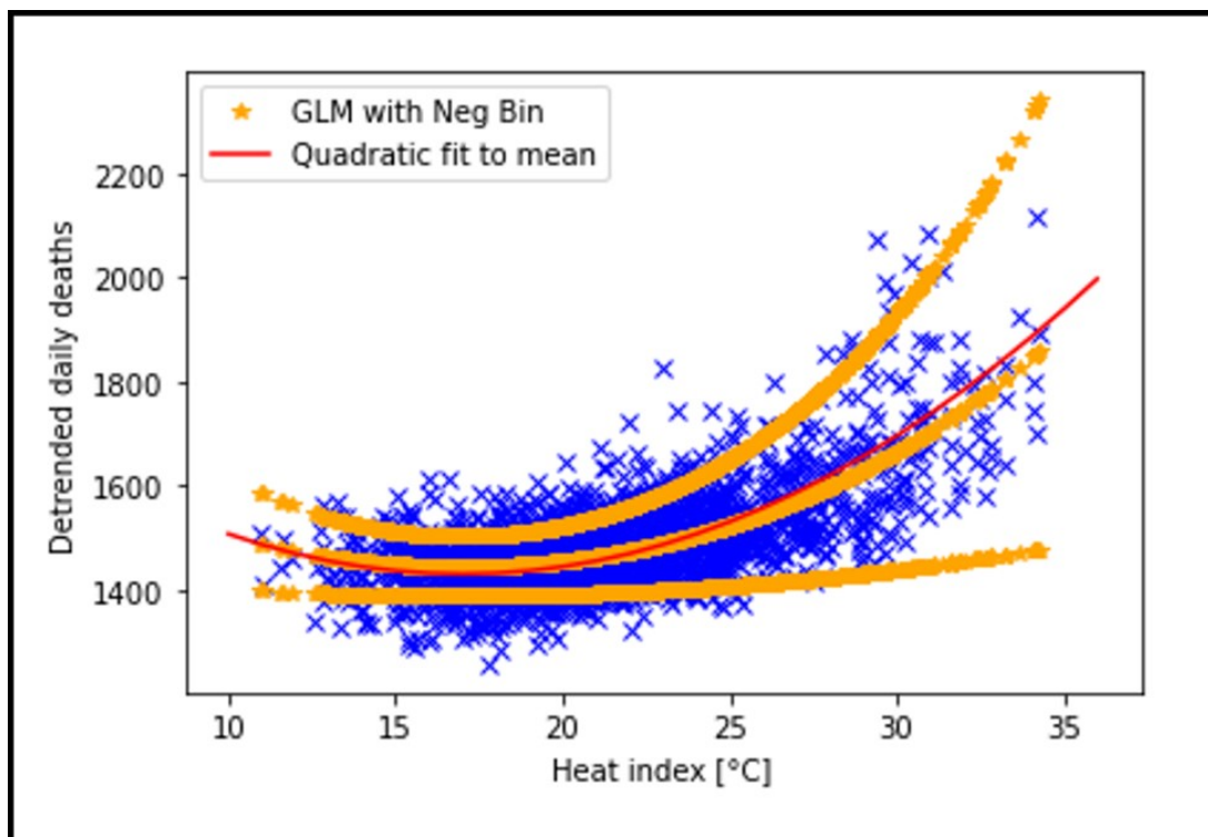
Figure 2.3. Polynôme déterministe du 2 me ordre (ligne rouge) et modèle linéaire généralisé (GLM) stochastique; distribution binomiale négative avec lien logarithmique (orange). Les courbes oranges donnent la meilleure estimation (courbe centrale) et bornes supérieures et inférieures de l'intervalle de confiance. En bleu le nombre de décès quotidiens en France en sus de la tendance vs l'Indice de Chaleur moyen en France, chaque jour durant les mois d'été, de 1970 à 1990. l'Indice de Chaleur provient des données ERA5 et le nombre de décès quotidiens en sus de la tendance provient de l'INSEE.
