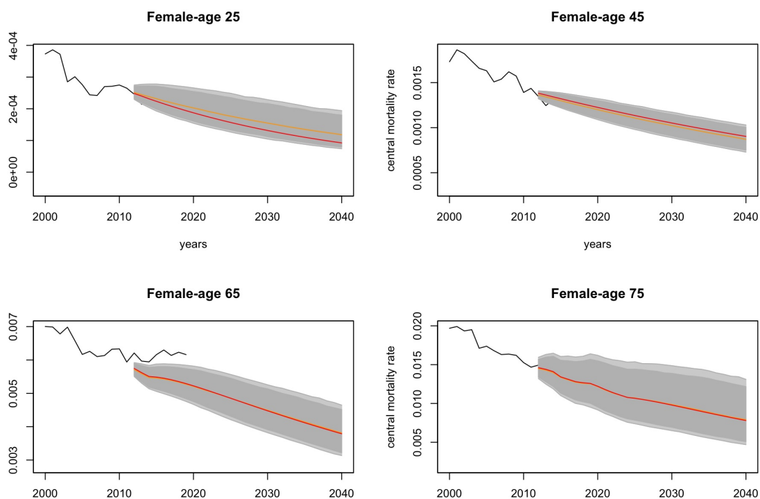
Figure 3.8. Taux de mortalité féminins projetés jusqu'en 2040, avec intervalles de confiance à 90% et 95% dans le scénario RCP2.6 (- : observé, - : prévision, - : trajectoire centrale des simulations).
