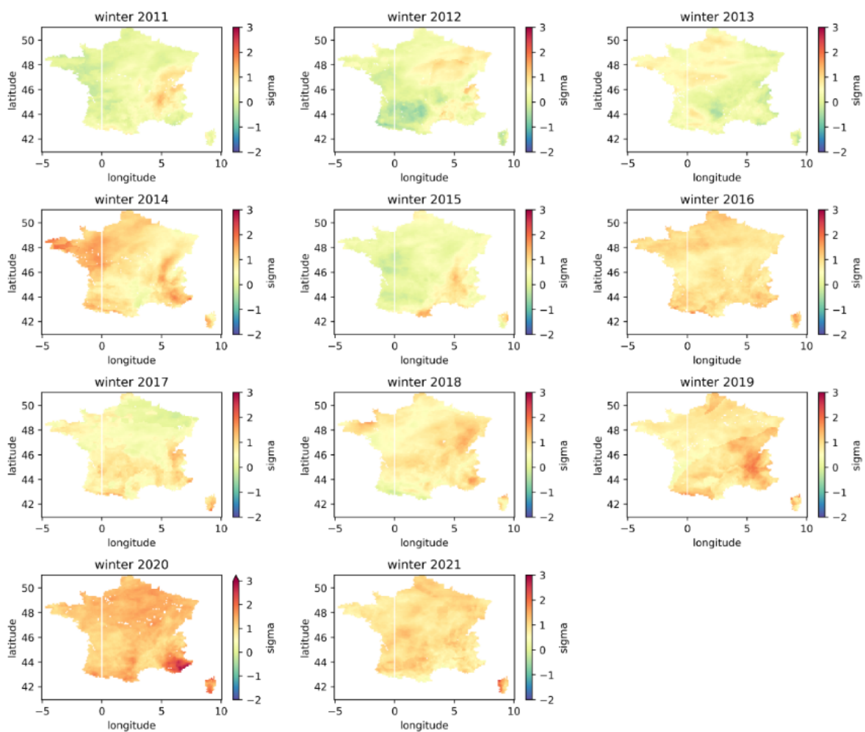
Figure A.1. Valeurs de l'ICAF l'hiver, 2011-2021.
