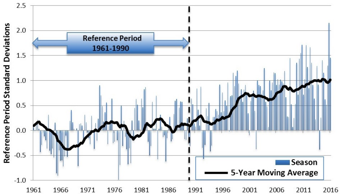
Figure 1.1. Valeurs de l'ACI de 1961 à 2021.
