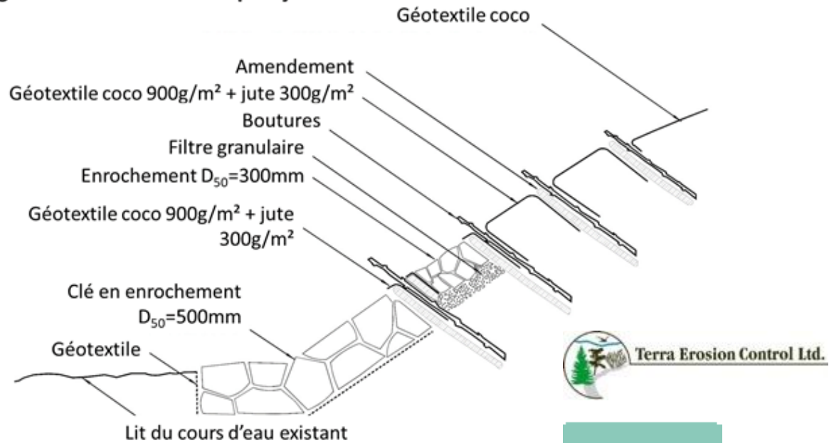
Profil type d'enrochement végétalisé avec clé et lit de plançons
