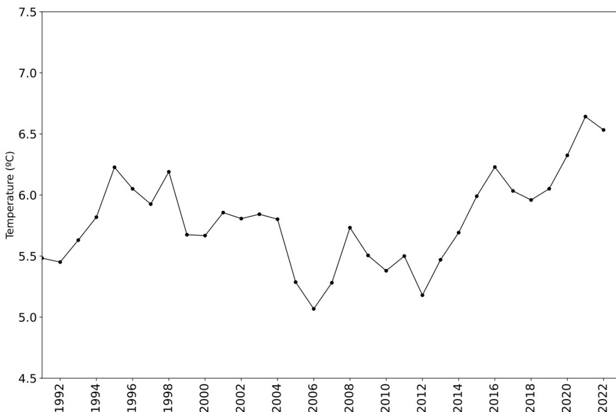
Figure 11 Températures moyennes annuelles (°C) à 140 m de profondeur au point B de 1991 à 2022
