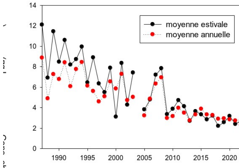
Figure 2 Evolution de la concentration moyenne estivale et annuelle en chlorophylle a ( \mu\text{g L}^{-1} ) dans la couche 0-18 m au point B de 1987 à 2022
