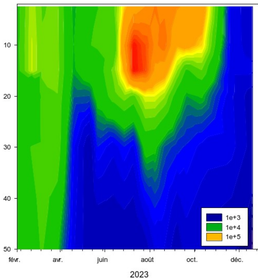
Figure 2: Distribution et dynamique des picocyanobactéries (en cellules / mL) en 2023 entre la surface et 50 m de profondeur dans le Léman à la station SHL2. L'échelle proposée est la suivante: 1e+3= 1000; 1e+4= 10000; 1e+5= 100000.
