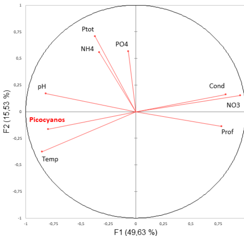
Figure 3: Analyse en composantes principales (ACP) effectuée avec quelques paramètres sur l'ensemble de l'année 2023, dans le Léman, à la station SHL2. La variance totale expliquée est de 65,2%.
