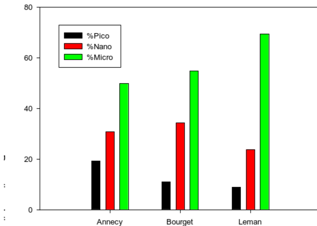
Figure 7: Evolution de la proportion (en %) de biomasse des compartiments pico-, nano- et microphytoplanctoniques dans les lacs Léman, d'Annecy et du Bourget pour la période 2014-2023.
