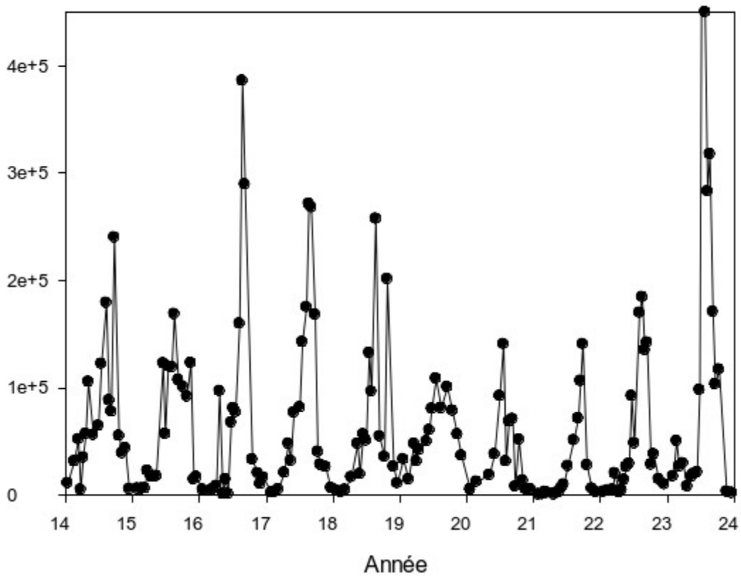
Figure 4: Evolution des concentrations moyennes de picocyanobactéries (en cellules/mL) entre 2.5 et 20 m de 2014 à 2023 inclus, dans le Léman, à la station SHL2.
