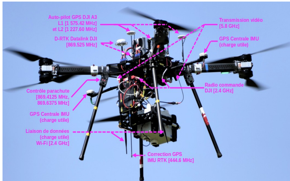
Fig. 1. - Système de communication du drone d'observation
