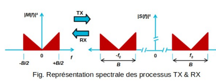
Fig. Représentation spectrale des processus TX & RX
