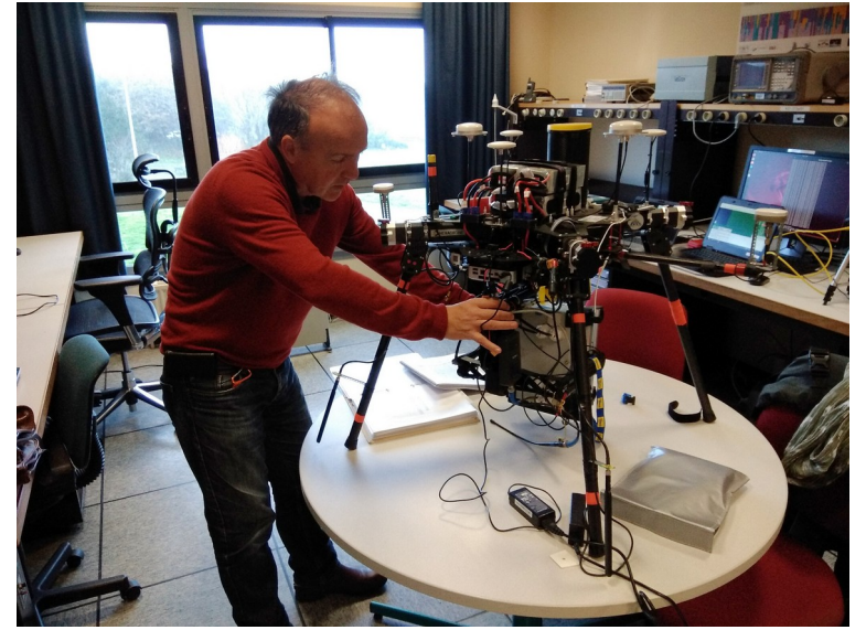
Fig. 2. - Préparation du drone pour l'analyse des signaux de radiocommunication
