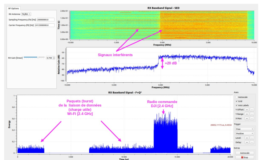
Fig. 6. - Application IHM d'analyse de spectre
