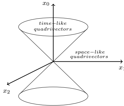
Fig 1 : Minkowski space
