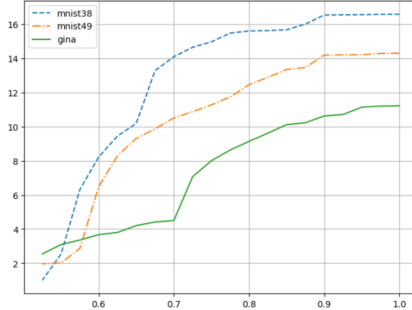
FIG. 3 – Taille moyenne des raisons \delta -probables lorsque \delta varie de 0, 5 à 1 (raisons suffisantes) pour les ensembles de données "mnist38", "mnist49" et "gina".
