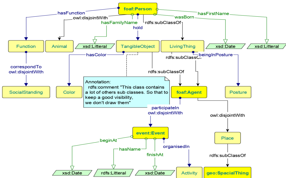
Figure 3 - Une vue de mediev'Enl avec ses super classes
