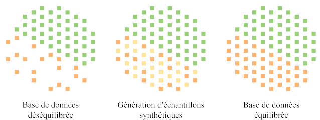
FIGURE 4 – Méthode SMOTE. En vert, la classe majoritaire. En orange, la classe minoritaire. En jaune, les échantillons synthétiques appartenant à la classe minoritaire.
