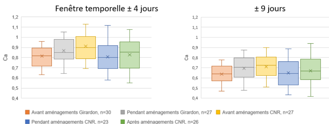
Figure 9. Evolution du coefficient de forme de crue à Beaucaire (scénario a)
