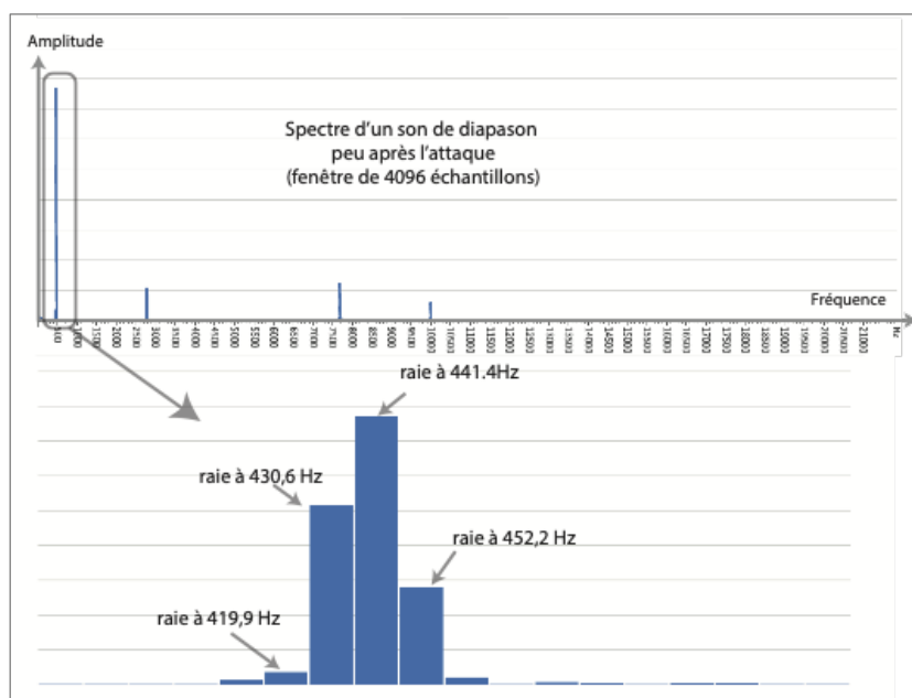
Figure 1. Spectre de raies obtenu par FFT d'un son de diapason (fenêtre de 4096 échantillons).
