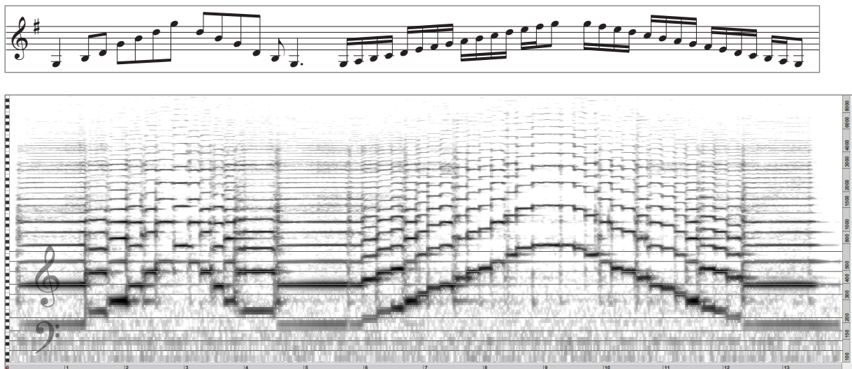
Figure 3. eE haut, une phrase de violon en notation traditionnelle ; en bas, le sonagramme de la même phrase de violon (durée : 13 secondes, logiciel Audiosculpt, fenêtres d'analyse de 4 096 échantillons).
