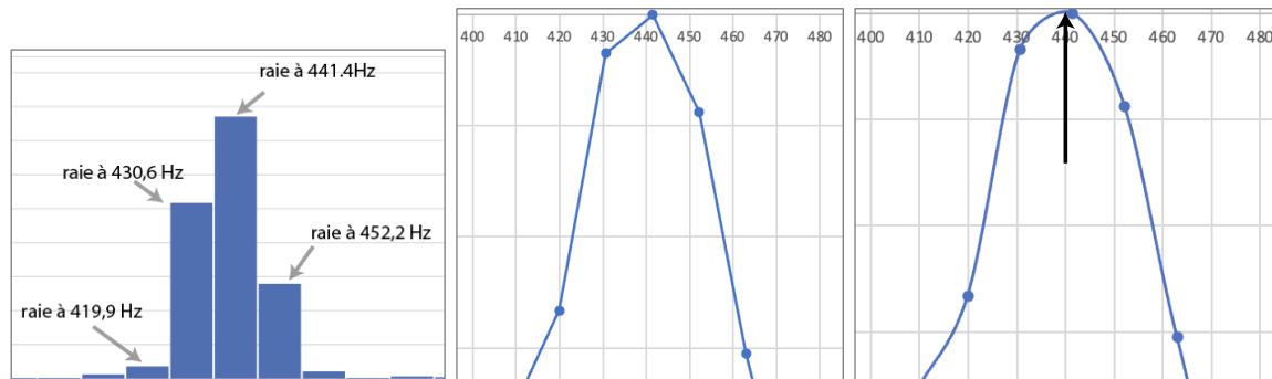
Figure 2. À gauche et au centre : quelques raies entourant un pic, valeur du pic : 441,4 Hz ; à droite : valeur estimée du pic : 440 Hz.
