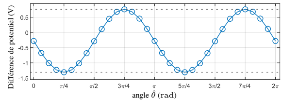
FIGURE 3. Différence de potentiels entre les électrodes de référence, e_1 et e_2 , et les électrodes de potentiels flottants, e_3 et e_4 , en fonction de l'angle \hat{\theta} entre l'aimant et le composite ME.
