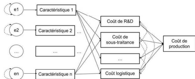
Figure 2. Structure générale du SEM du coût estimé
