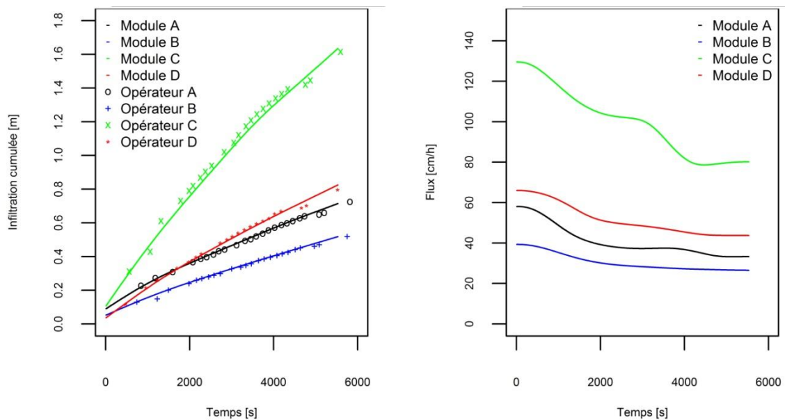
Figure 7. Evolution de l'infiltration cumulée et du flux au cours du temps.
