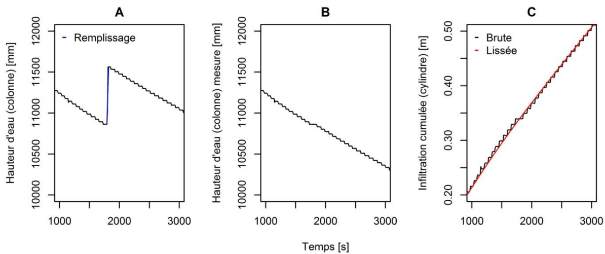
A : données brutes – B : suppression des phases de remplissages – C : infiltration cumulée brute et lissée
