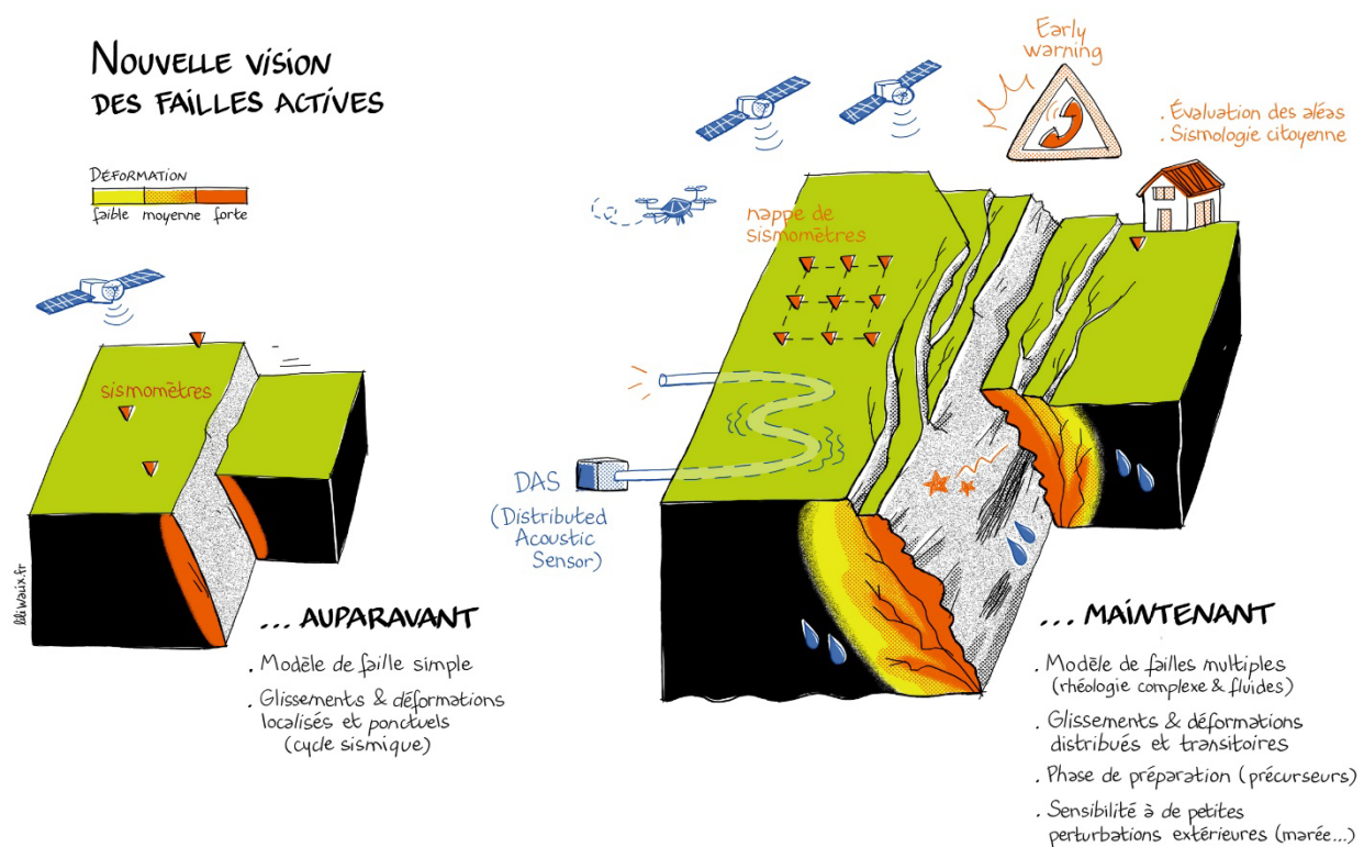
Figure 2. Un changement majeur dans la conceptualisation des failles actives a émergé grâce à une intensification et une diversification des mesures de terrain et à des avancées marquantes en modélisation et analyse des données. La zone impliquée dans le cycle sismique est beaucoup plus distribuée, avec un réseau complexe de failles intriquées qui peut s'étendre lors de l'endommagement engendré par le séisme et dont le glissement est activé non seulement lors de la rupture mais aussi lors de la déformation lente du milieu tout au long du cycle sismique (figure de droite). Cette nouvelle vision génère des questions clés : Quel est le rôle des déformations lentes du milieu dans le bilan d'énergie global lié au cycle sismique ? Quels sont les impacts en termes d'aléas ? Quel est le mode opératoire de cette déformation aismique hors et sur les failles ? Quel est le rôle de la circulation des fluides ? Comment améliorer la détection des événements et la mesure de l'évolution 4D du système ? Comment calculer les impacts sur les bâtis et contribuer à l'alerte précoce ?
