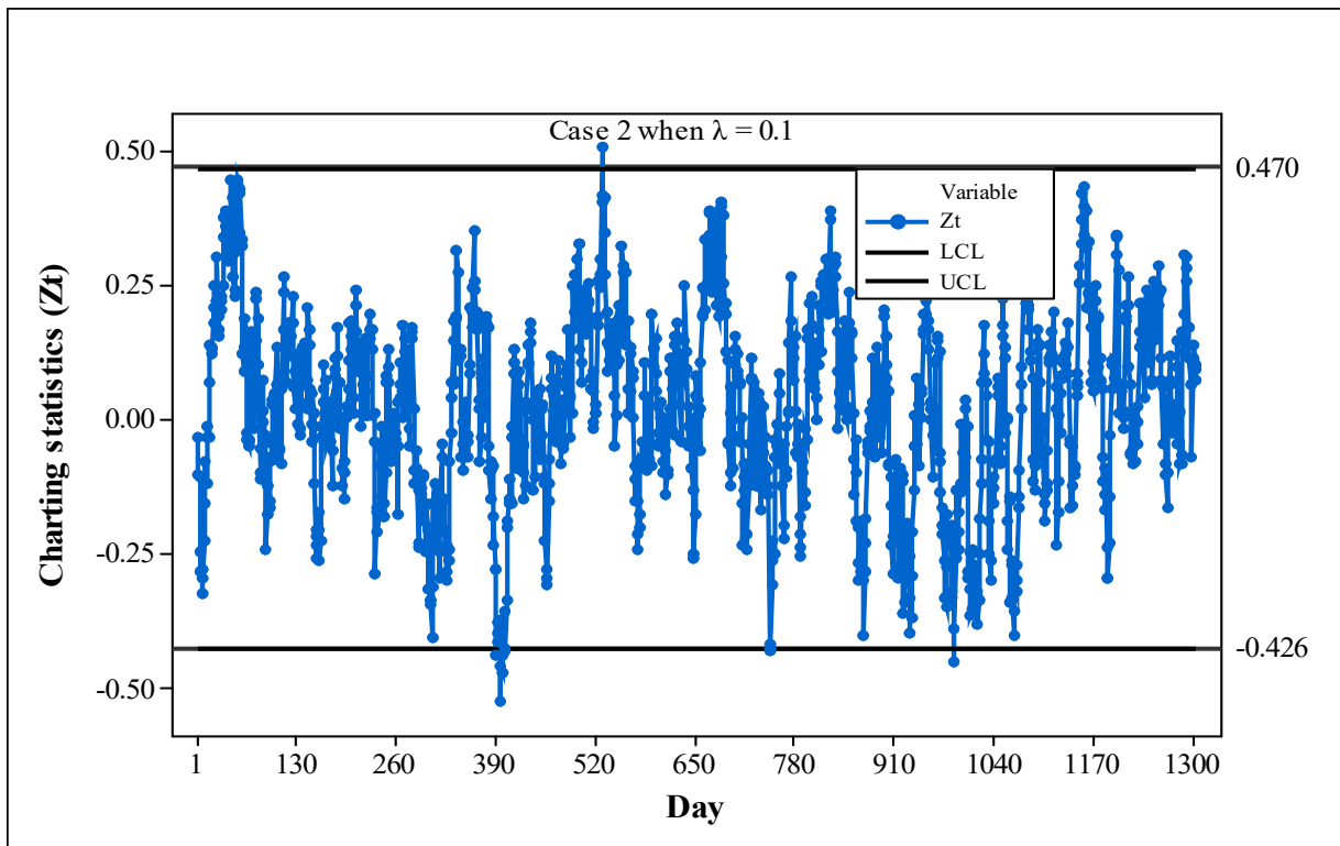
(d) Case 2 when \lambda = 0.1 (OOC 393 rd sample)
