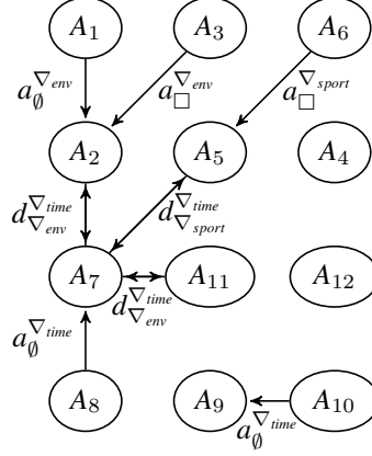
Fig. 3. Argumentation graph
