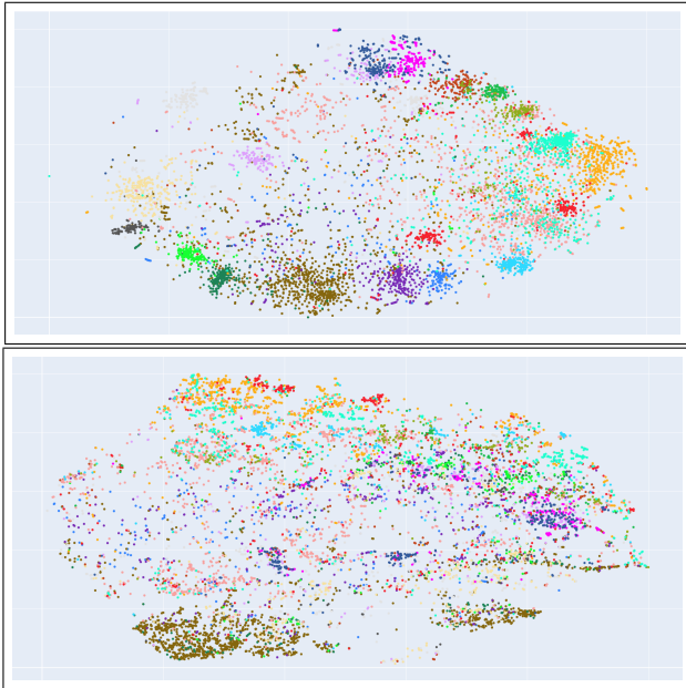
FIGURE 3 – Visualisation t-SNE des vecteurs des 20 nouvelles classes (1 couleur = 1 classe) obtenus par a) Resnet101 entraîné sur ImageNet (module PCB) b) Yolov8 entraîné sur les 60 classes de base seulement.
