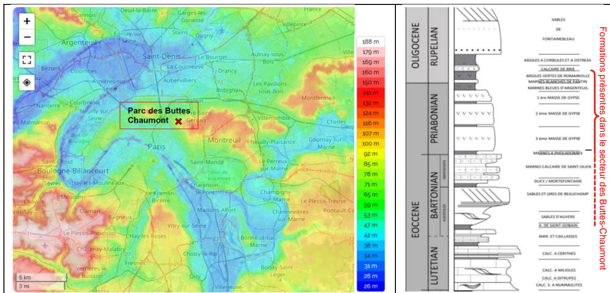
Figure 1. Contexte topographique du parc et coupe géologique associée (Briais, 2015)
