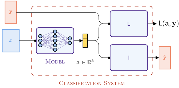
FIGURE 1 – Illustration d’un système neuronal de classification
