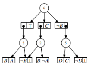
FIGURE 3 – Représentation graphique d'un SDD dans [12]
