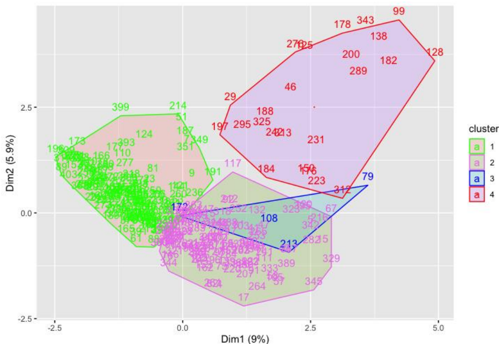
Figure 2: Quatre profils identifiés grâce aux méthodes d'analyses multifactorielles et de classification
