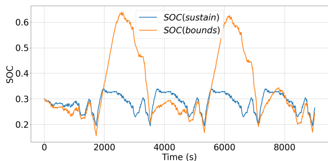
FIG. 7. Évolution du SOC pour chaque stratégie
