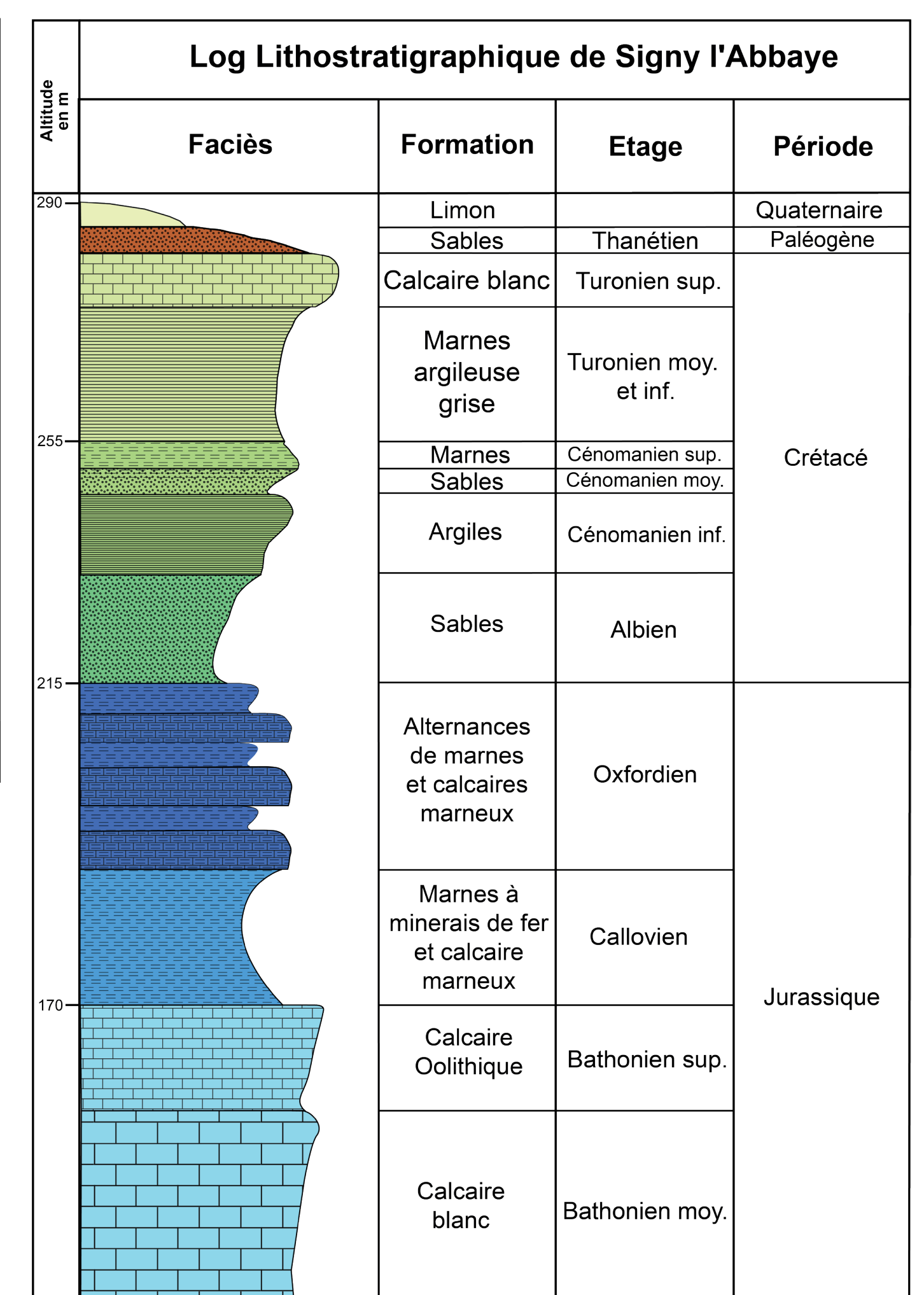
Fig. 3 log lithostratigraphique de Signy-l'Abbaye
