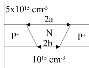
Fig.7 : Schéma du canal d'un JFET pour la détermination de l'angle de gravure
