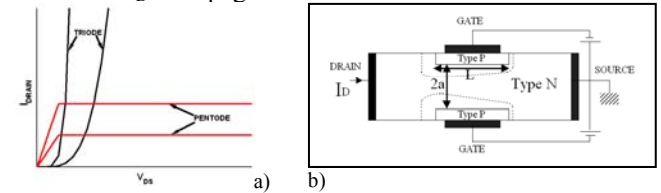
Fig. 3 : Formes des caractéristiques électriques des JFET (a) et vue en coupe d'un transistor JFET élémentaire (b) avec ses paramètres L , 2a et la limite de charge d'espace
