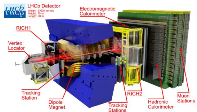
Figure 2 – Composition du détecteur LHCb
