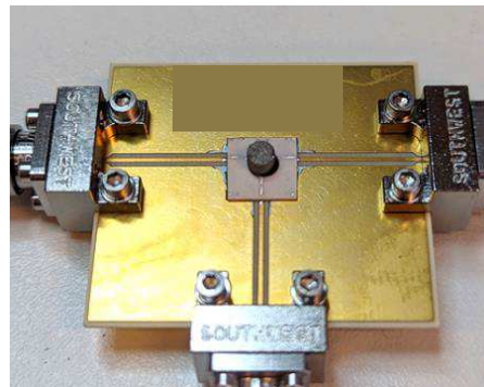
Figure 8. Circulateur reporté
