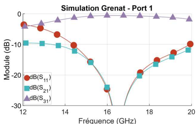
Figure 4. Simulation du circulateur sur Grenat
