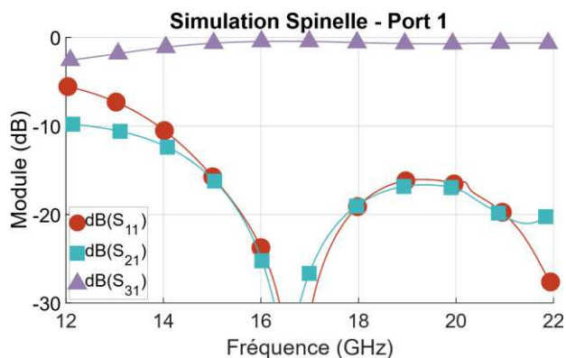
Figure 5. Simulation du circulateur sur Grenat
