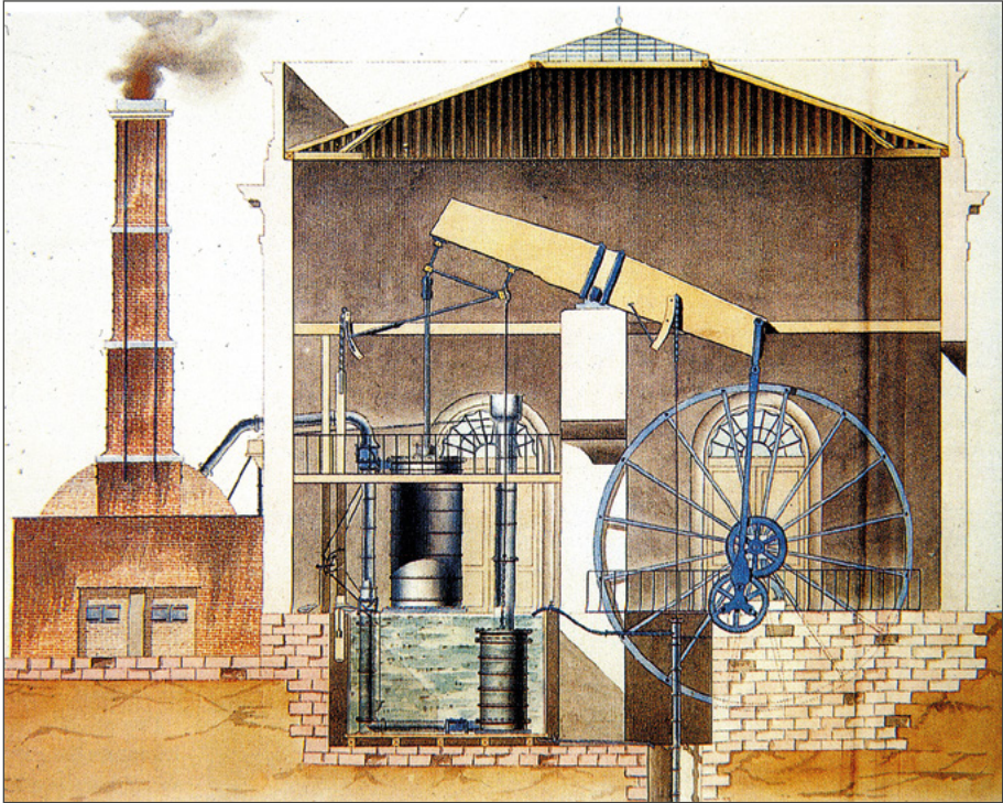
Figure 1. Fragment du dessin de la machine à vapeur à double effet par A. Betancourt, 1789, par Gouzévitch (photo 1). © École des Ponts et Chaussées. FA. Ms 104/2 : Navigation intérieure. Machines, 1784 - 1790.
