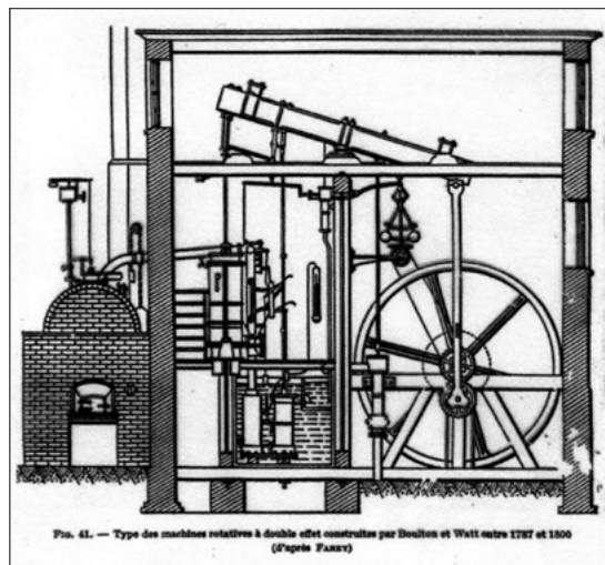
Figure 3. Fragment de la copie du dessin de la machine à vapeur de Watt (1787-1800) reconstruite et publiée pour la première fois, dans J. Farey, (1827), A treatise on the steam engine, historical, practical, and descriptive (XIII, [2], 728 p., XXV f. de pl. [Plate XI]), Longman, Rees, Orme, Brown, and Green.
