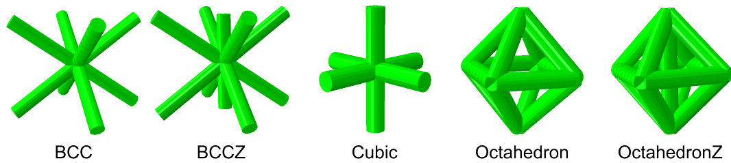
FIGURE 2 – Cellules élémentaires représentatives des structures lattices étudiées.
