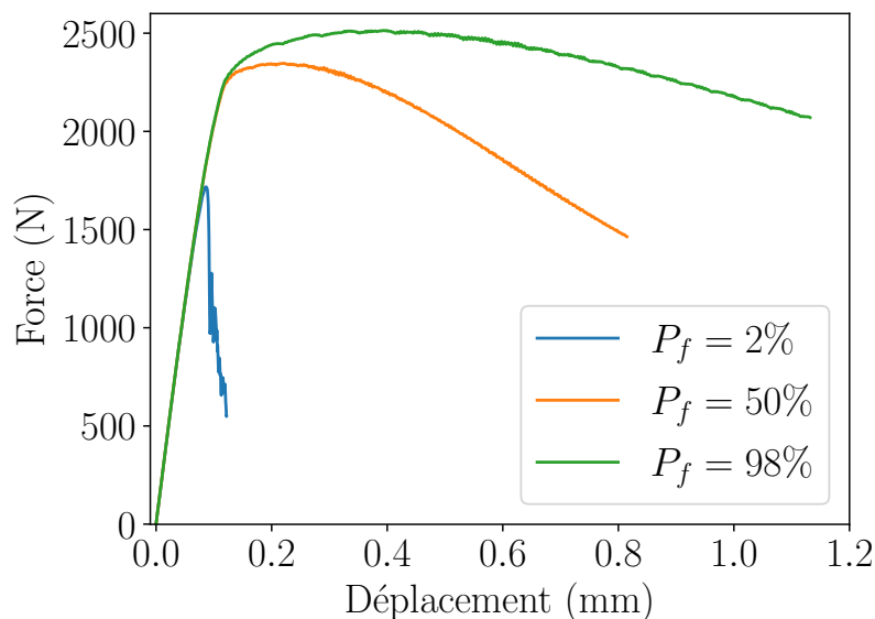
FIGURE 6 – Courbes force-déplacement obtenues par simulation à -120^\circ\text{C}
