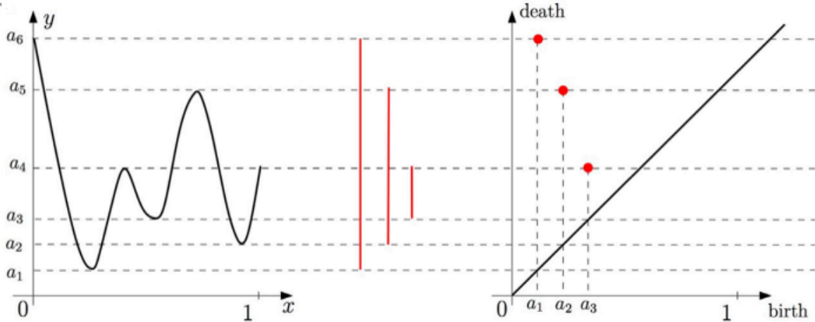
FIGURE 2 – Exemple d’une fonction f : [0, 1] \rightarrow \mathbb{R} (à gauche), de son code-barre (au milieu) et son diagramme de persistance (à droite). Tiré de [10]
