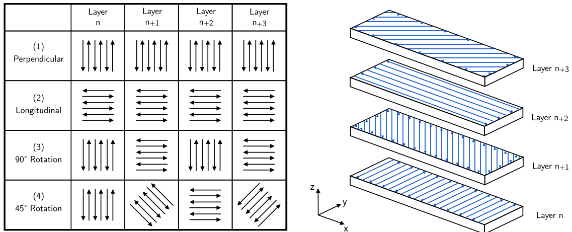
FIGURE 2 – Exemples de stratégies de lasage possibles [11].
