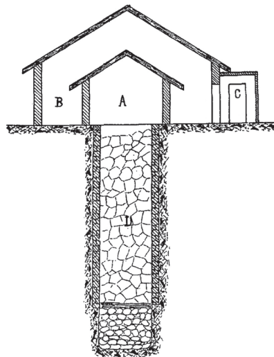
Fig. 76. — Glacière industrielle.
