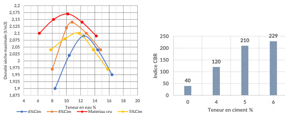
FIGURE 7. (a) Courbes montrant l'évolution de la densité OMP en fonction de la teneur en ciment (b) Evolution de l'indice CBR du mélange avec la teneur en ciment
