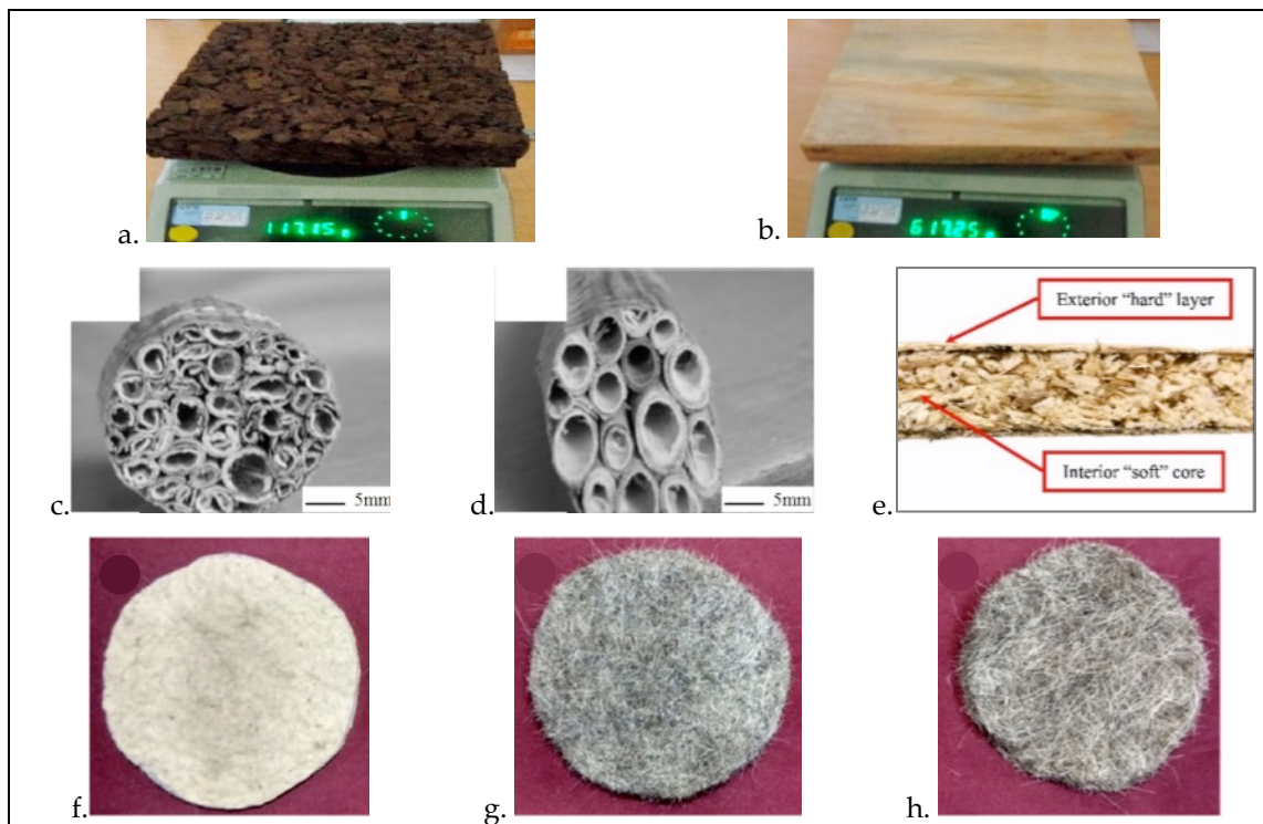
FIGURE 3. Panneau d'écorces de chêne (a) et de pin massif (b) (Limam et al., 2016), bottes d'orge (c) et de roseaux (d) (Véjélienè et al., 2011), vue en coupe d'un panneau de rachis de maïs (e) (Platt et al., 2023), laines de mouton (f), de chèvre (g) et crin de cheval (h) (Ahmed et al., 2019).
