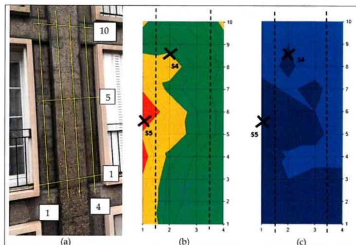
FIGURE 5. Exemple de diagnostic (étage 2 – poteau intermédiaire- potentiel vs AG/AgCl (mV) et Résistance en \kappa\Omega réalisés par la ville du Havre (dossier ville)
