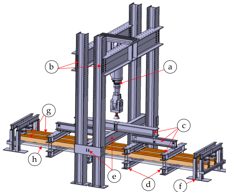
Figure 3. (a) Vérin hydraulique, (b) Portique, (c)-(d) Système de chargement, (e) Système de guidage, (f) Système d'appui, (g) Poutres en bois, (h) Dalle de béton.
