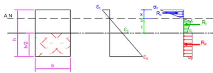
FIGURE 12. Schémas de calcul de la répartition des déformations et des contraintes dans une section à deux couches au moment de la formation de fissures.
