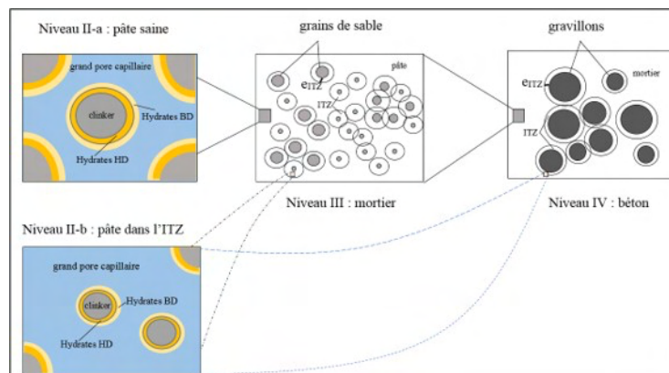
Figure 1 – Modèle multi-échelle de prédiction des propriétés diffusives du béton (Achour et al. 2020).
