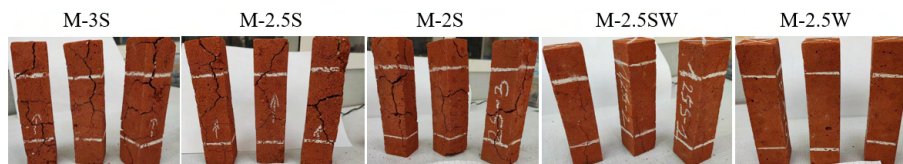
FIGURE 4. Faciès de rupture des éprouvettes après le cycle chauffage/refroidissement de 800°C.
