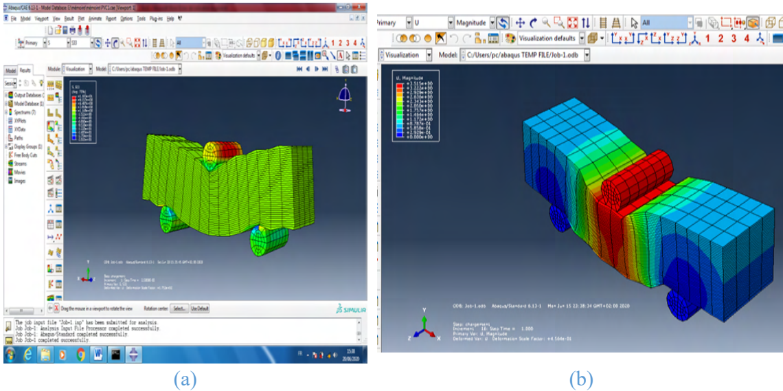
FIGURE 4. Modèle numérique de modélisation des mortiers.
