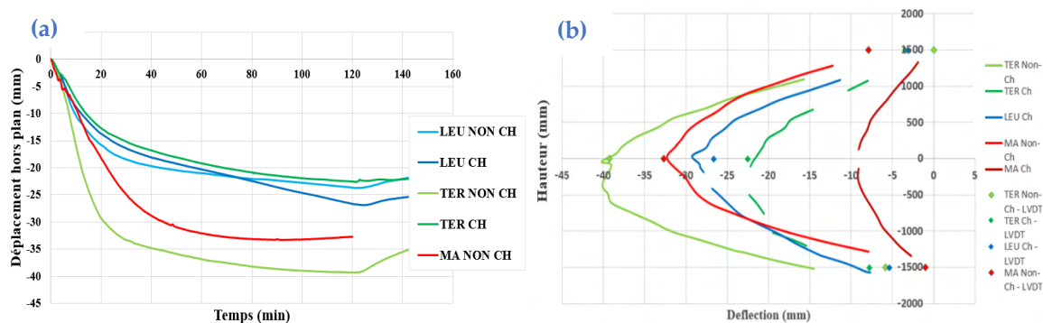
FIGURE 4. (a) L'évaluation du déplacement hors-plan obtenu par LVDT au centre du mur pendant le chauffage dans les murs ; (b) Profils de déformation le long de la hauteur à mi-largeur des murs à la fin du chauffage par les résultats des LVDTs et la DIC
