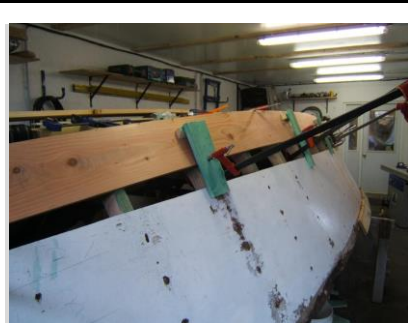
Ill. 5. Changement du bordé en contre-plaqué en bordé à clins. © Alain Cormier, Stéphane Perrin, 2015.
